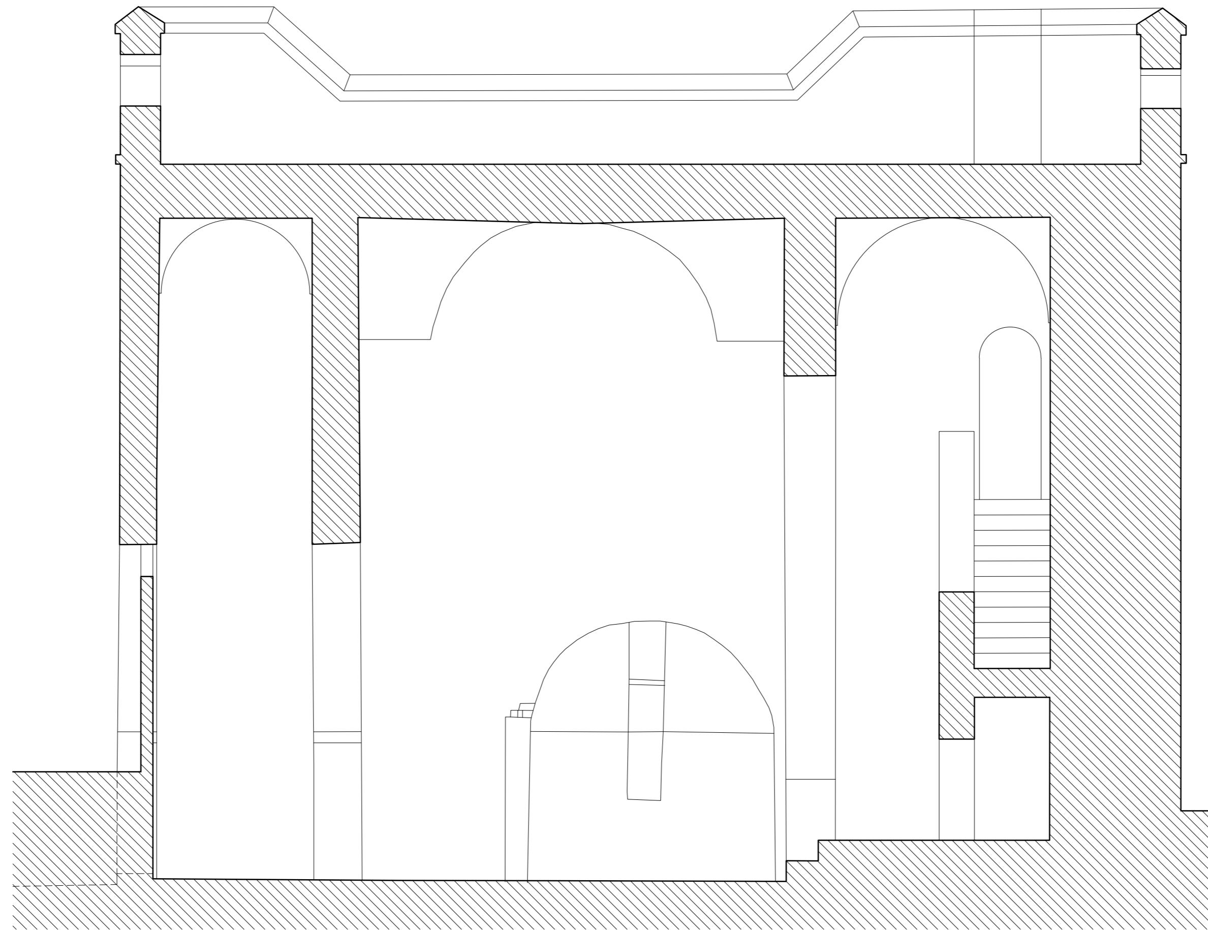
0 5 10 m BAB AYLAN. MARRAKECH A. ALMAGRO / arq. RABASF SECCION NOVIEMBRE 2018
