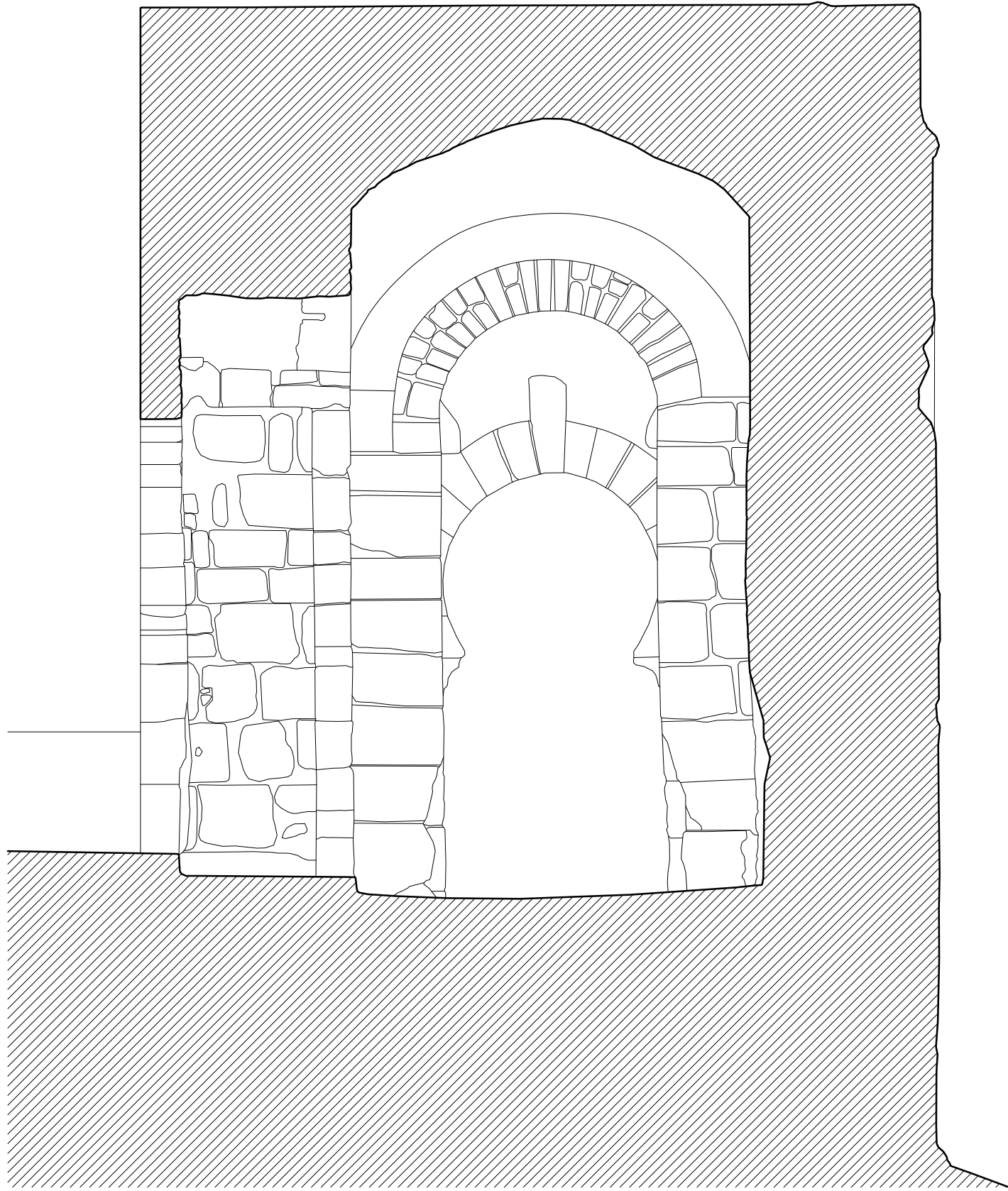
SECCION NORTE- SUR HACIA ESTE
