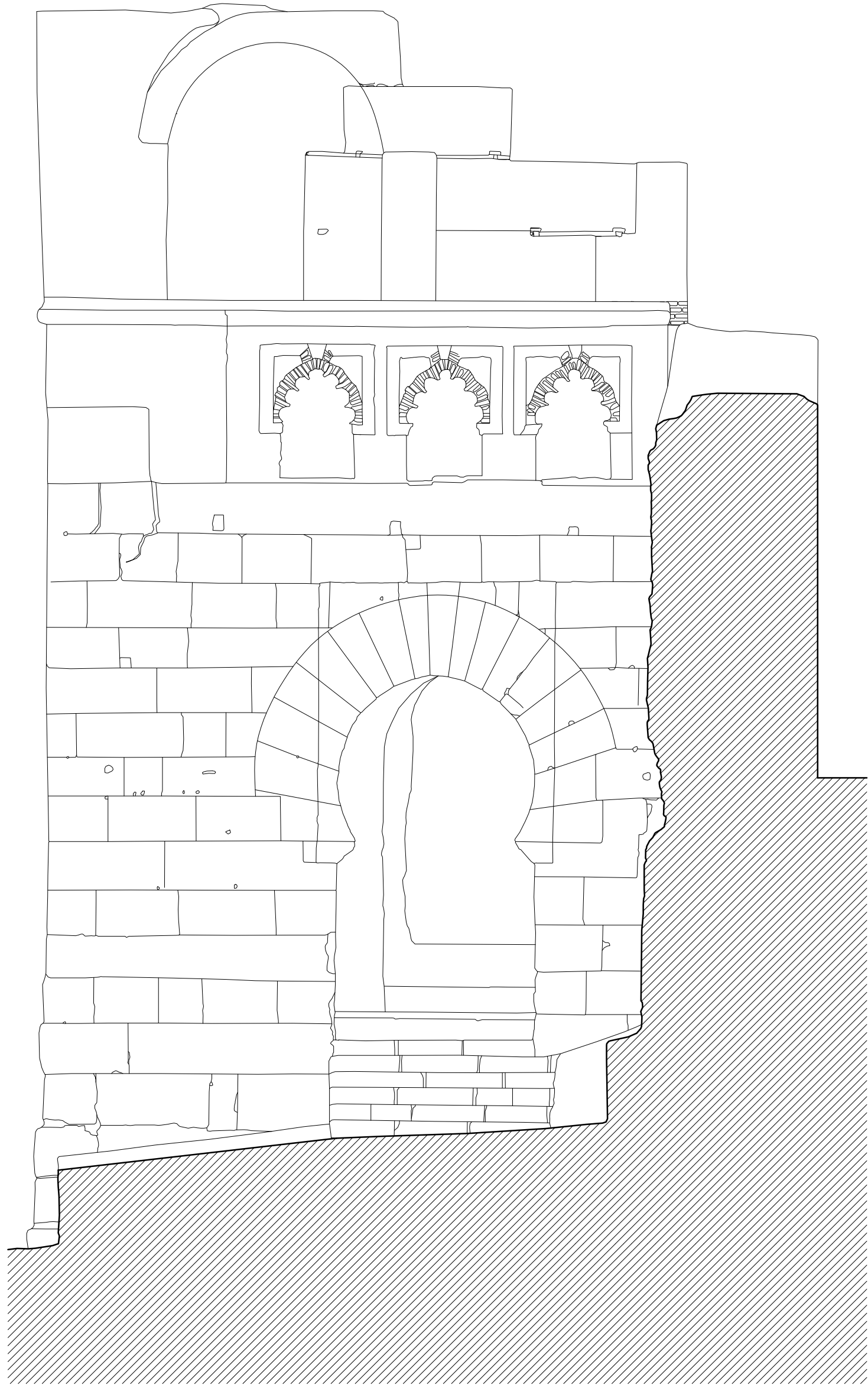
ALZADO ESTE
