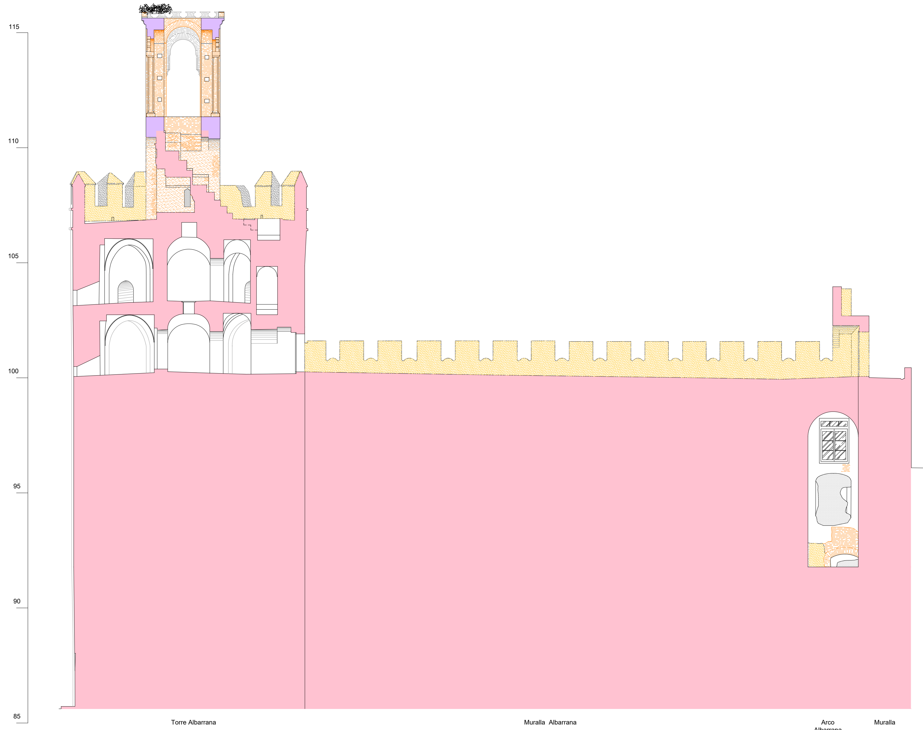
SECCIÓN LONGITUDINAL
