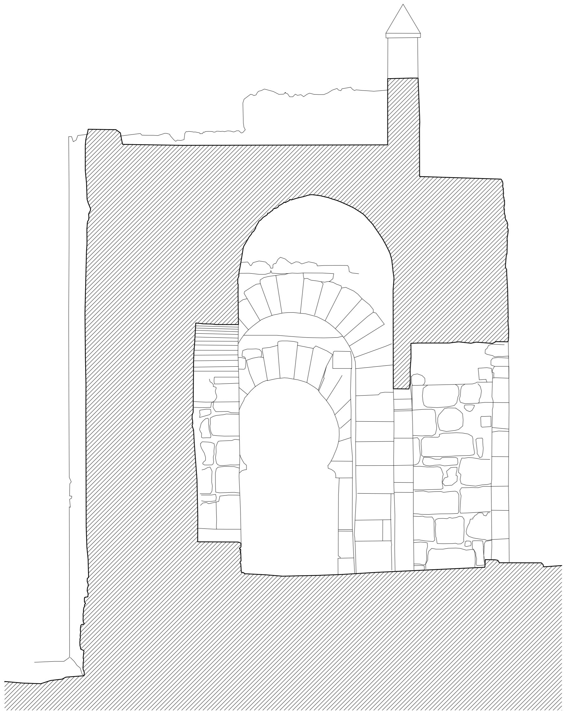
SECCION O-E
