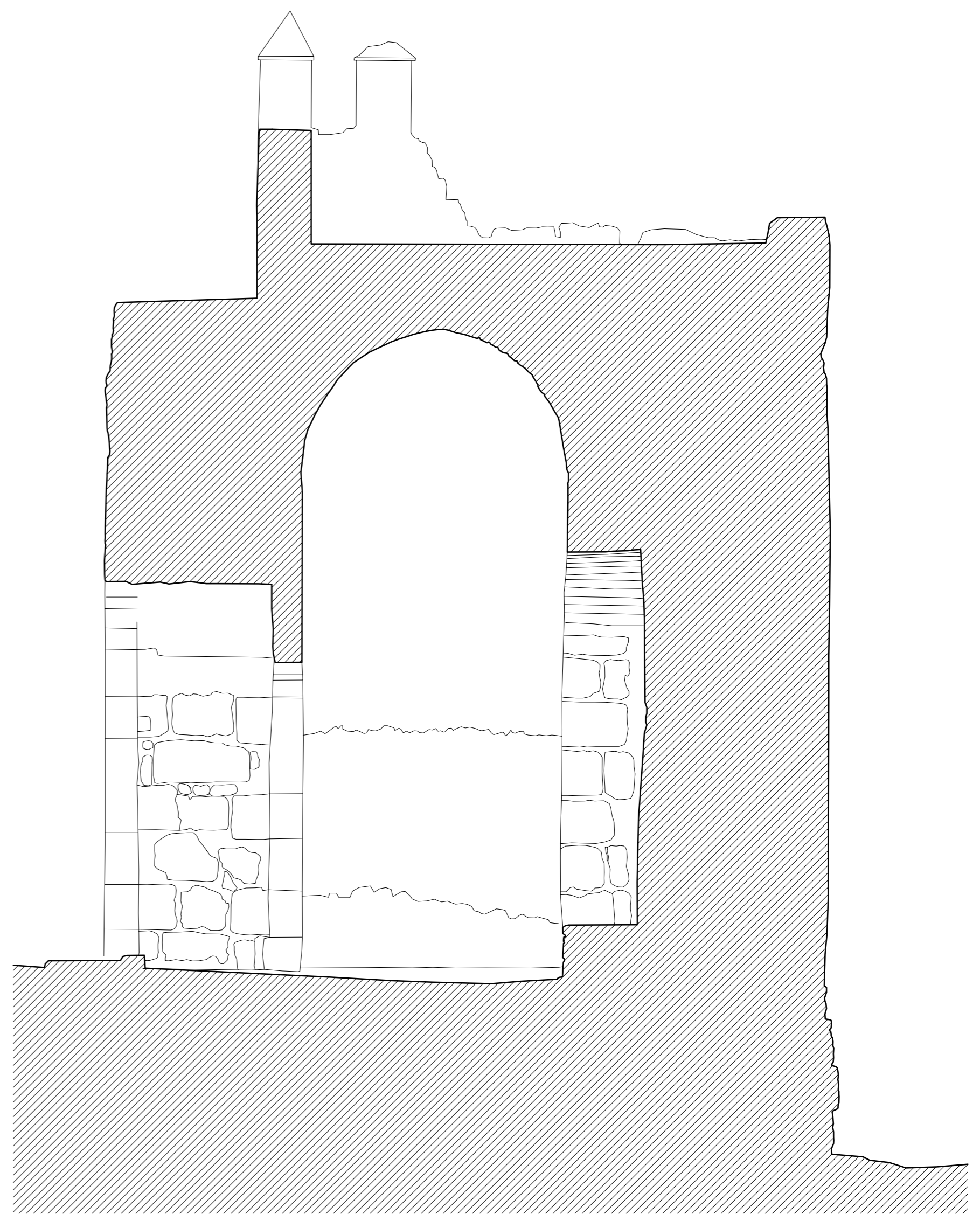
SECCION E-O
