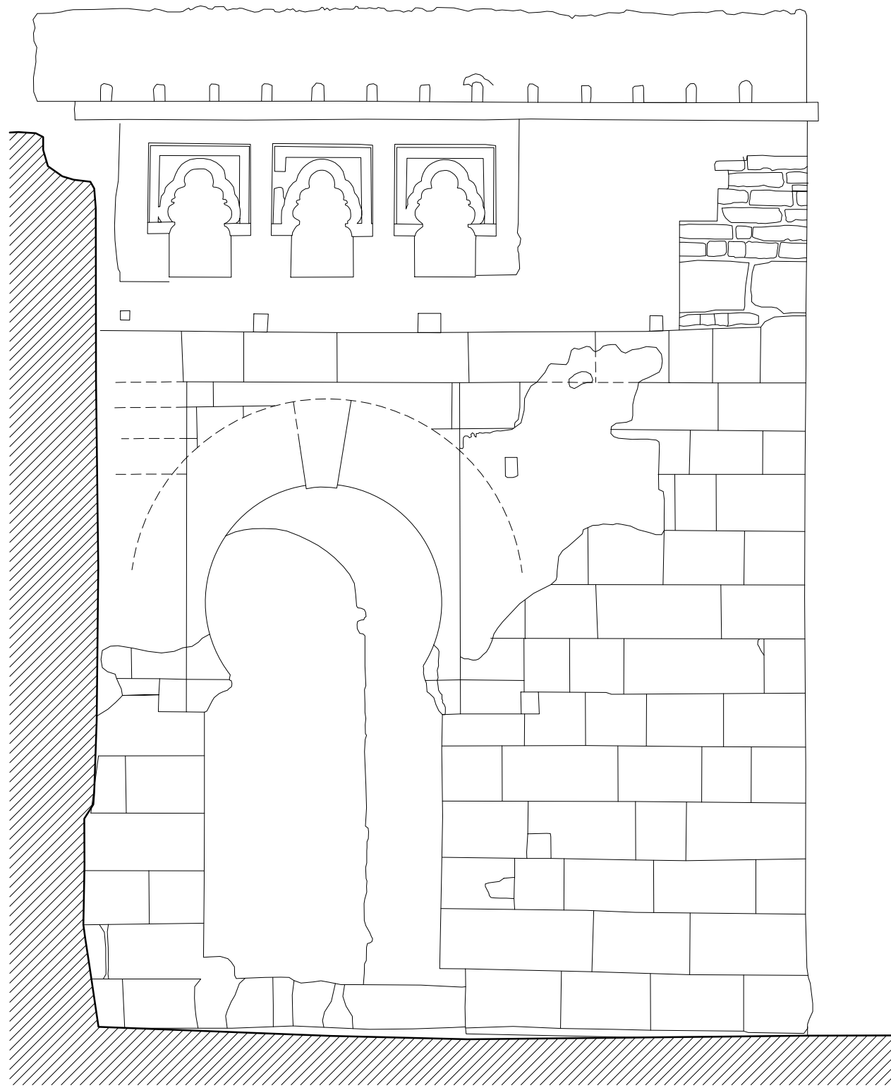
ALZADO ESTE (EXTERIOR)
