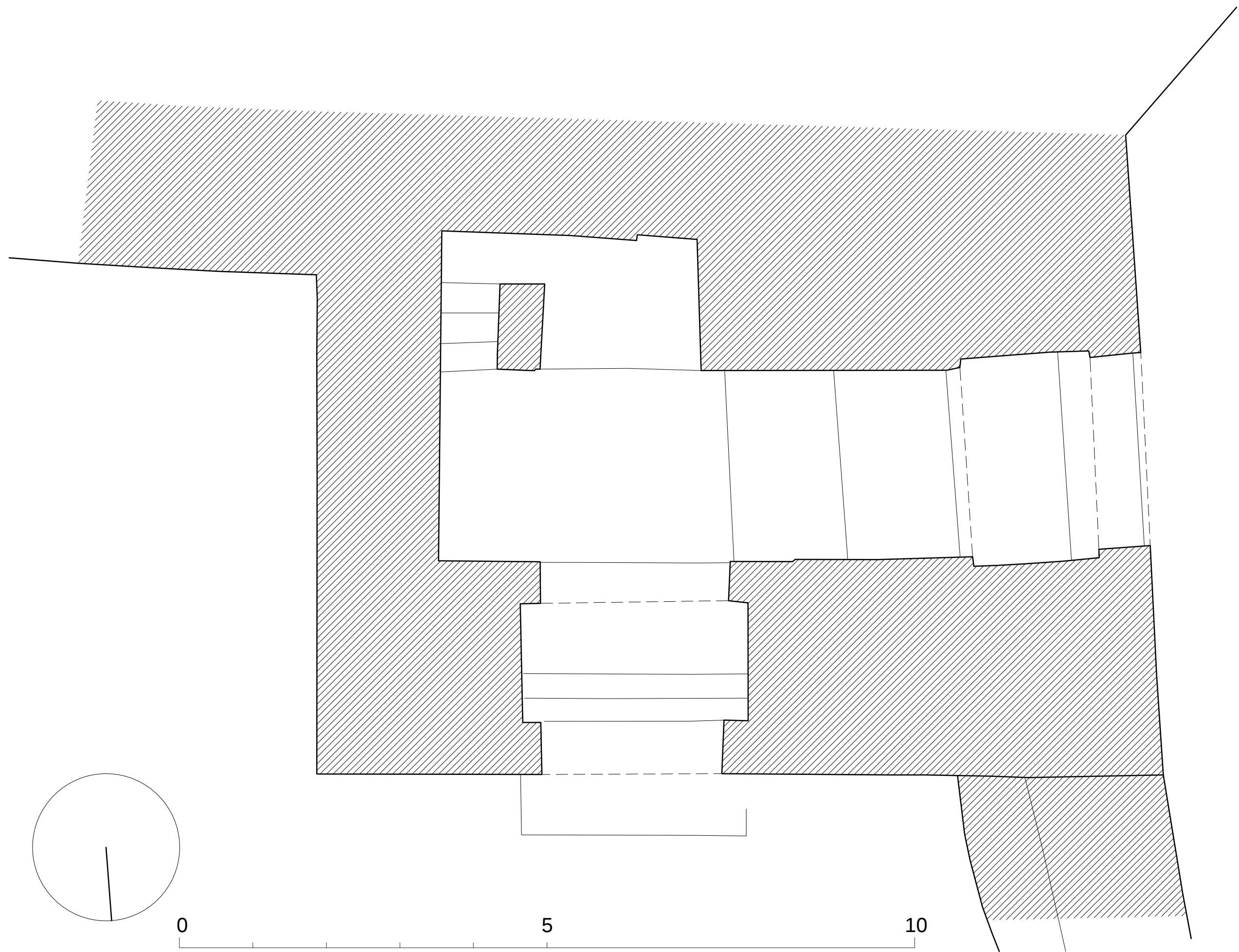
BAB YAMA'A DEL RECINTO AMURALLADO DE TAZA (MARRUECOS) A. Almagro e I. Almela / arqs. RABASF UNED febrero 2025
