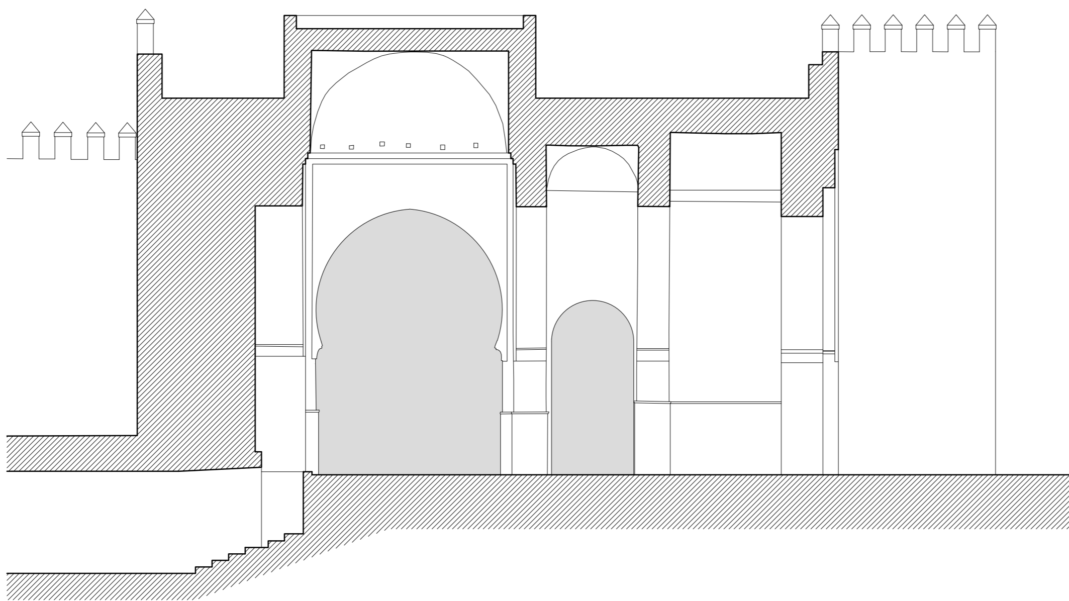
SECCIÓN B
