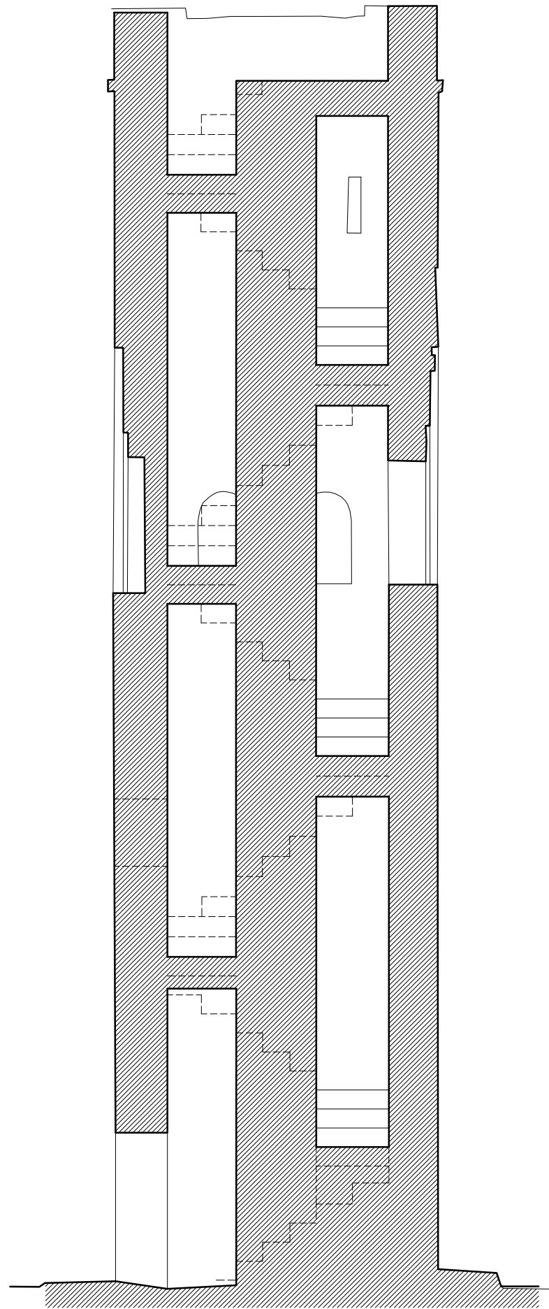
SECCION OESTE- ESTE
