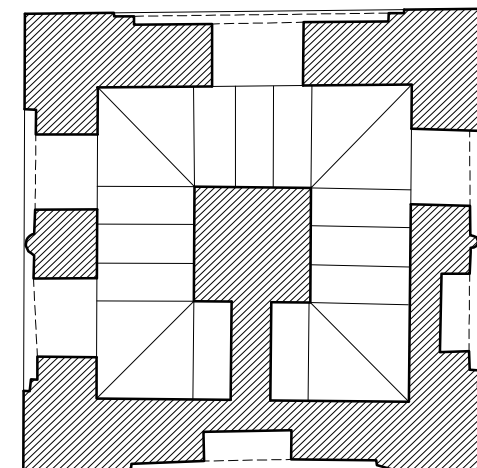
PLANTA SUPERIOR
