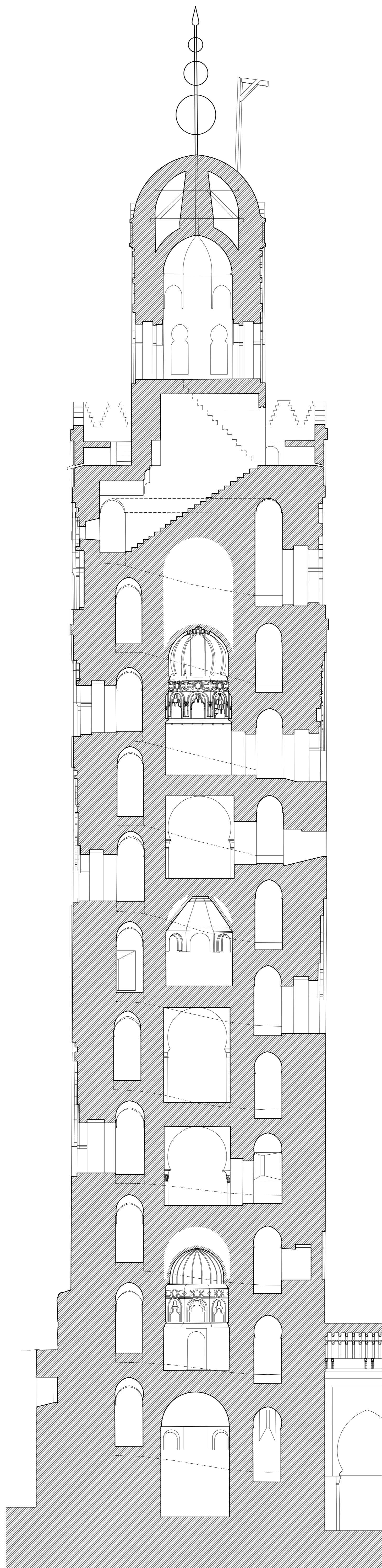
0 5 10 m ALMINAR DE LA MEZQUITA KUTUBIYYA DE MARRAKECH ESQUELETO DE ESTUDIOS ANIMÉS S.L. - 1999 2013 - A. ALMADRERA
