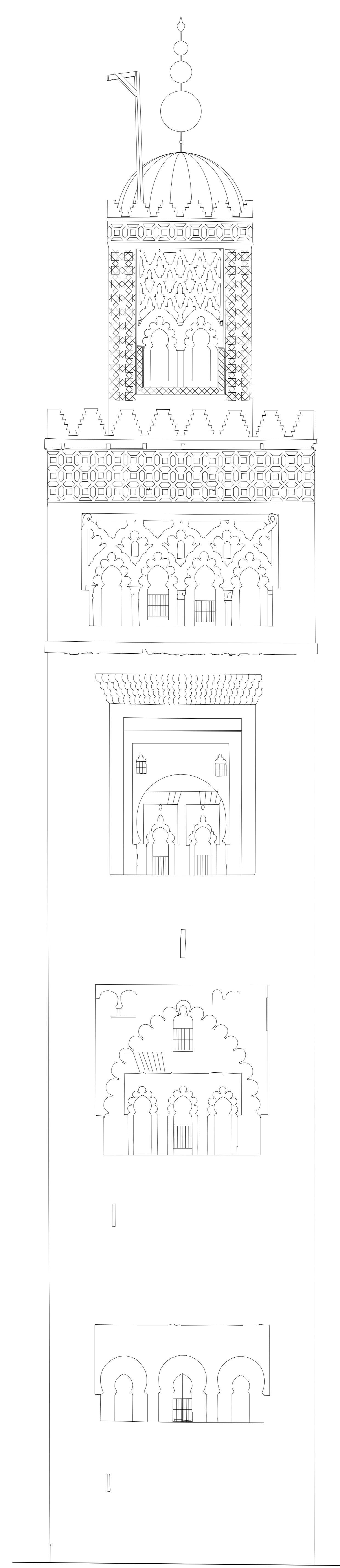
ALZADO ESTE
