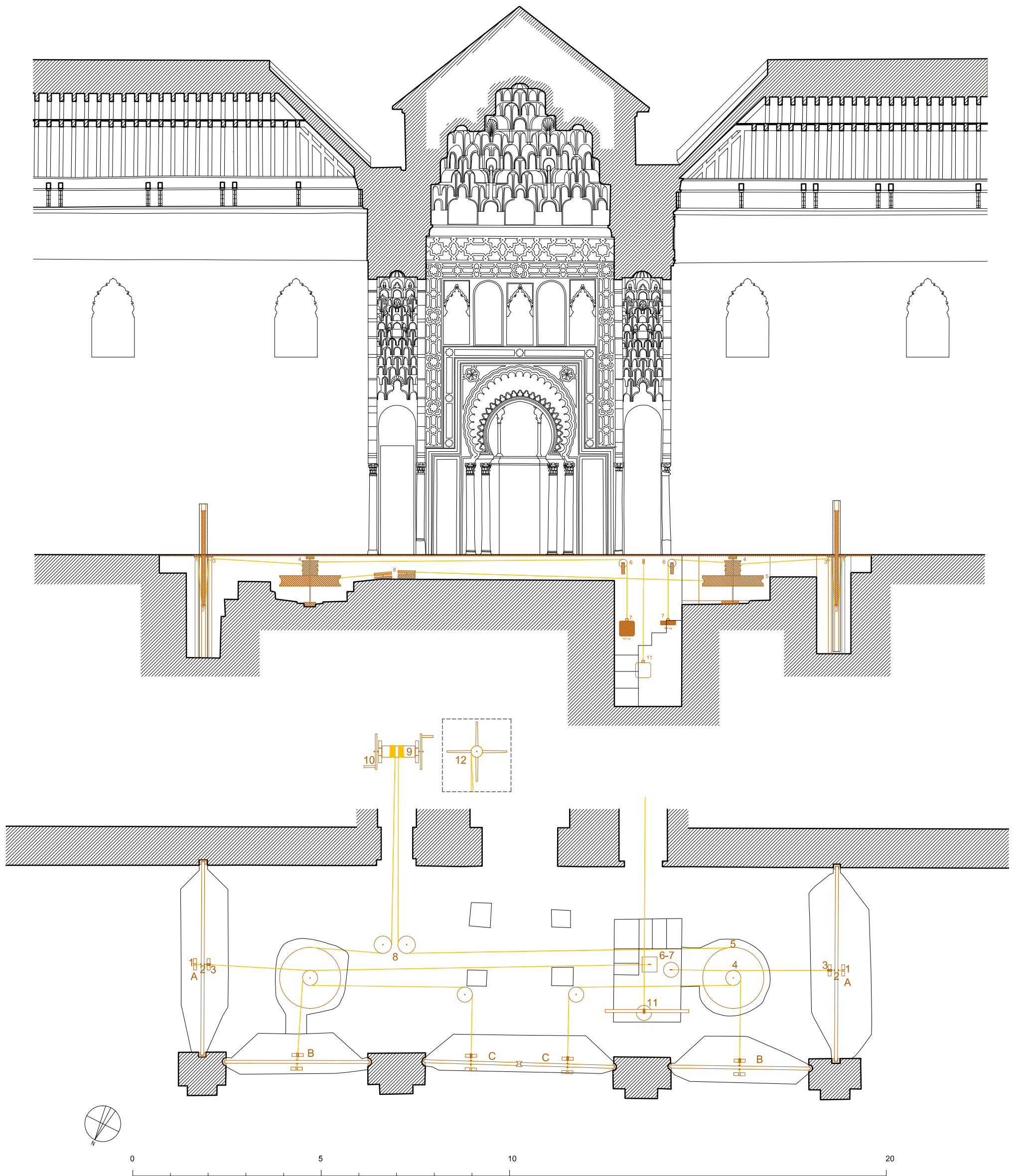
MEZQUITA KUTUBIYYA DE MARRAKECH. AREA DE LA MAQSURA. HIPÓTESIS
