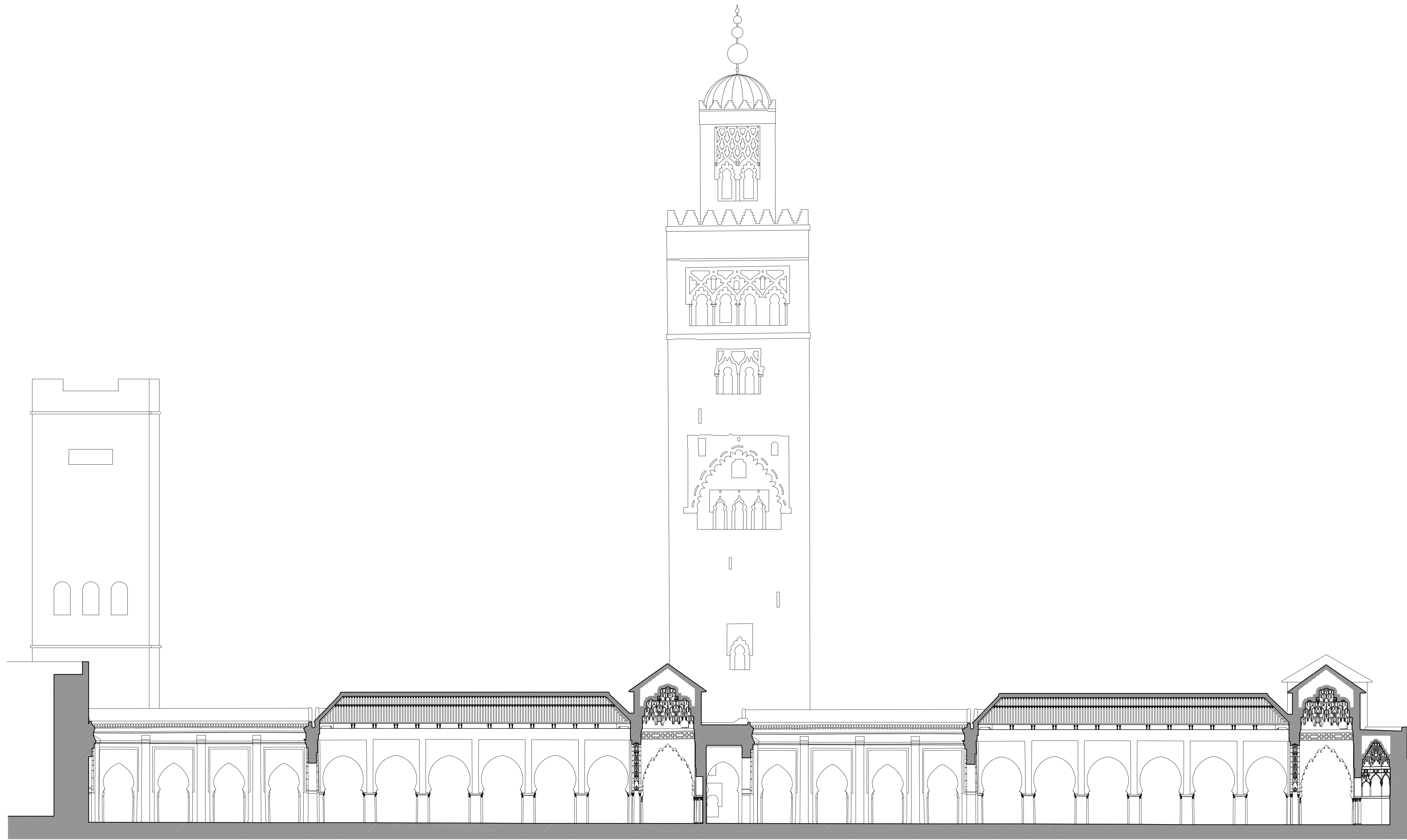
MEZQUITA KUTUBIYYA DE MARRAKECH. SECCIÓN LONGITUDINAL POR EL MIHRAB A. ALAMORFI IFIG. ESCUELA DE ESTUDIOS ÁRABES, CSIC, GRANADA ENERO 2011
