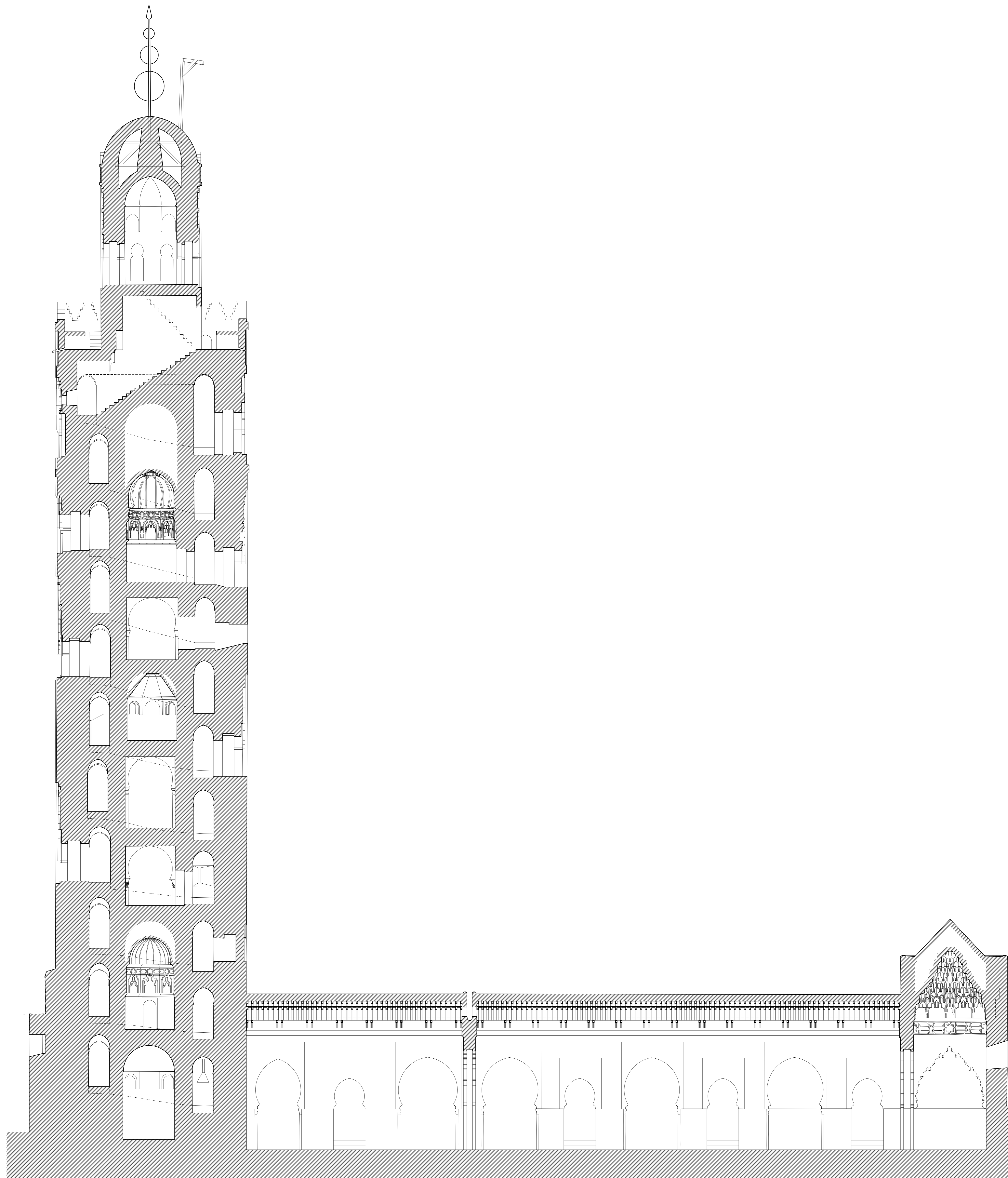
MEZQUITA KUTUBIYYA DE MARRAKECH. SECCIÓN LONGITUDINAL POR EL ALMINAR Y LA SALA DE ORACIÓN A. ALMAGRO | ARQ. ESCUELA DE ESTUDIOS ÁRABES, CSIC, GRANADA ENERO 2018
