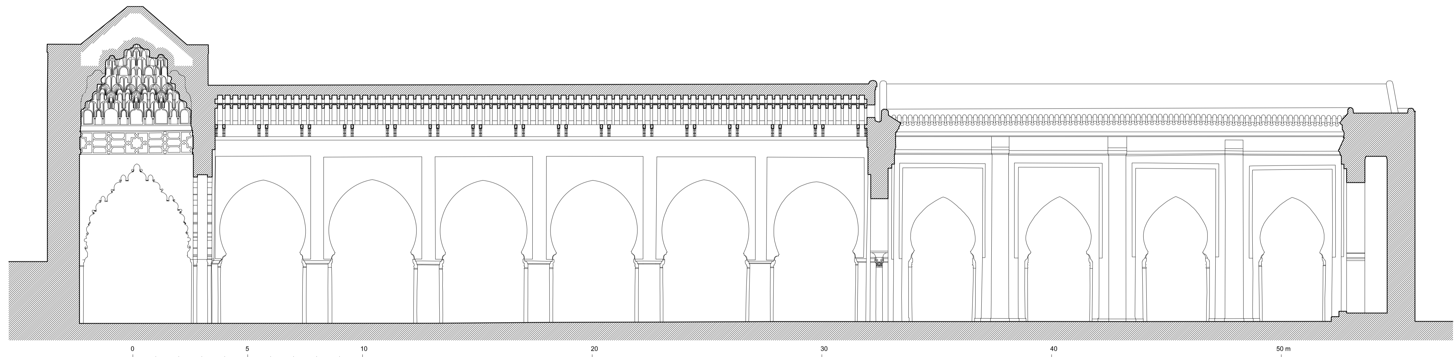
MEZQUITA KUTUBIYYA DE MARRAKECH. SECCIÓN LONGITUDINAL POR LA SALA DE ORACIÓN A. ALMAGRO / ARQ. ESCUELA DE ESTUDIOS ÁRABES. CSIC. GRANADA ENERO 2018
