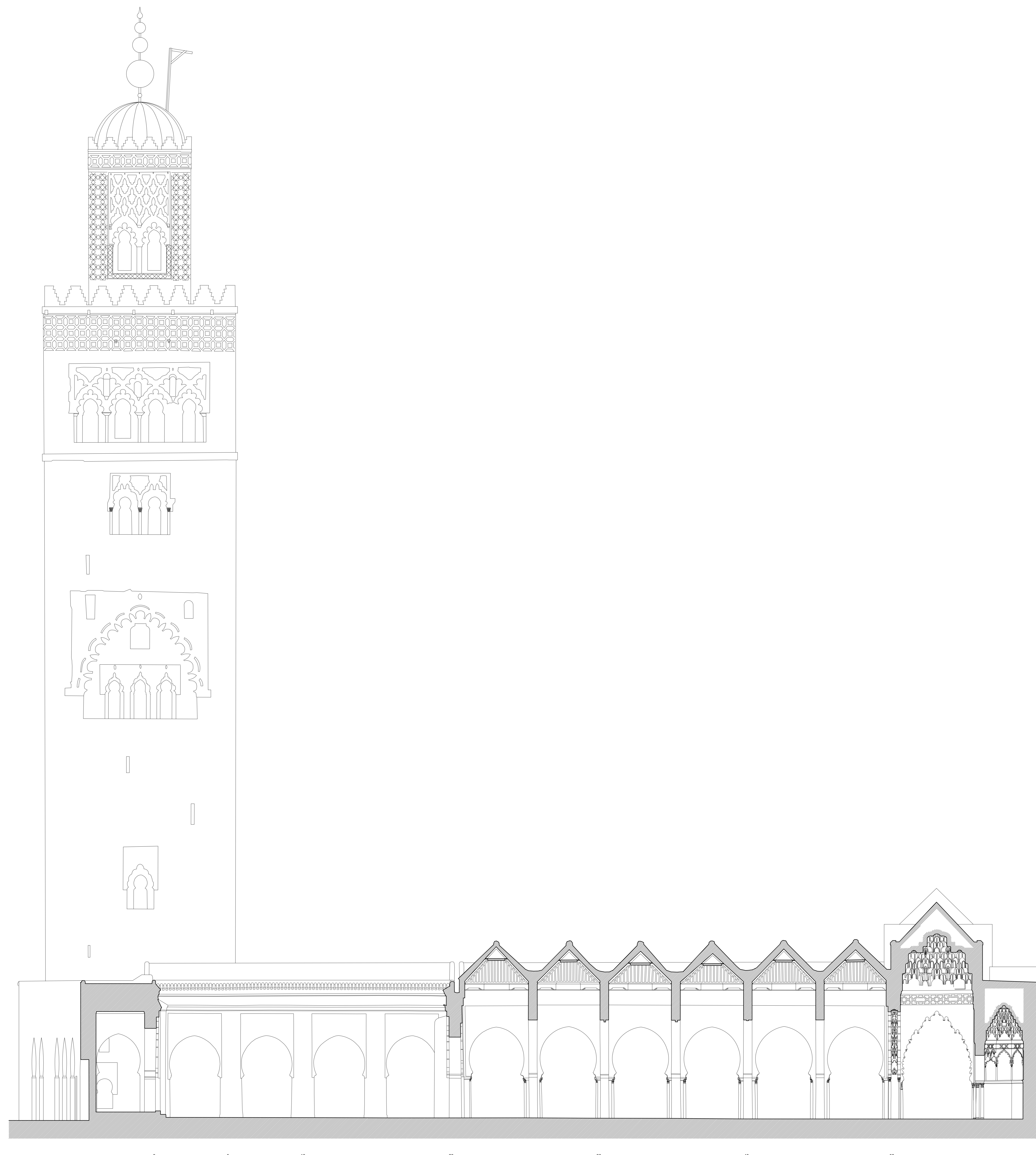
MEZQUITA KUTUBIYYA DE MARRAKECH. SECCIÓN LONGITUDINAL POR EL MIHRAB A. ALMAGRO / ARQ. ESCUELA DE ESTUDIOS ÁRABES, CSIC, GRANADA ENERO 2018
