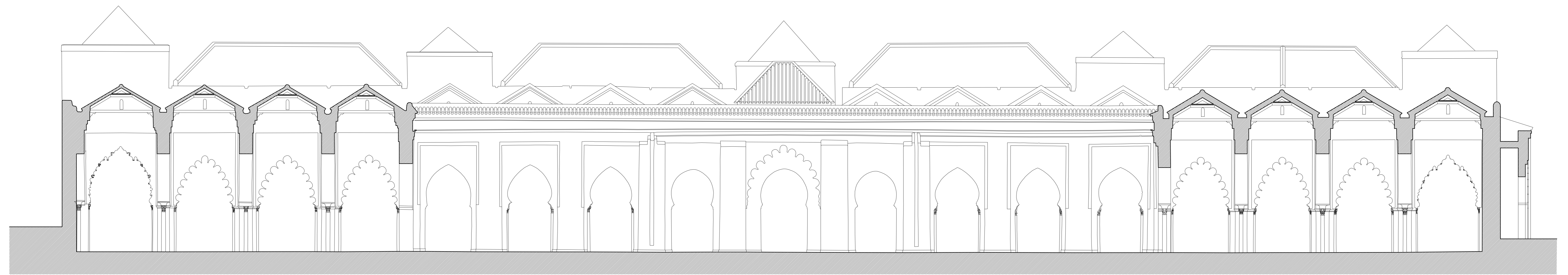
MEZQUITA KUTUBIYYA DE MARRAKECH. SECCIÓN TRANVERSAL POR EL PATIO A. ALMAGRO | ARG. ESCUELA DE ESTUDIOS ÁRABES, CSIC, GRANADA ENERO 2018
