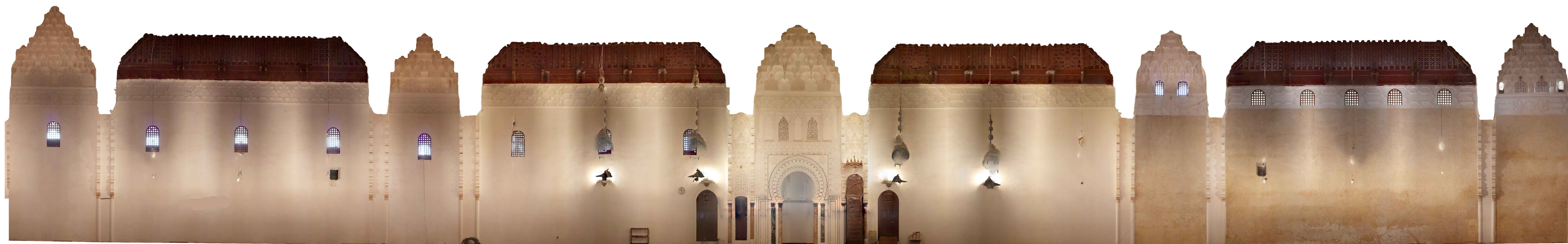
MEZQUITA KUTUBIYYA DE MARRAKECH. SECCIÓN TRANSVERSAL POR LA NAVE DE LA QIBLA A. ALMAGRO / ARO, ESCUELA DE ESTUDIOS ÁRABES, CSIC, GRANADA ENERO 2016
