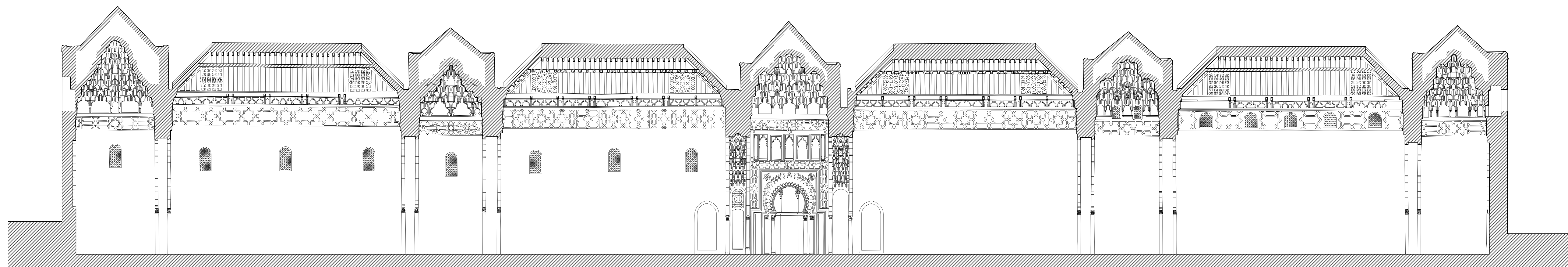
MEZQUITA KUTUBIYYA DE MARRAKECH. SECCIÓN TRANSVERSAL POR LA NAVE DE LA QIBLA A. ALMAGRO / ARO, ESCUELA DE ESTUDIOS ÁRABES, CSIC, GRANADA ENERO 2016
