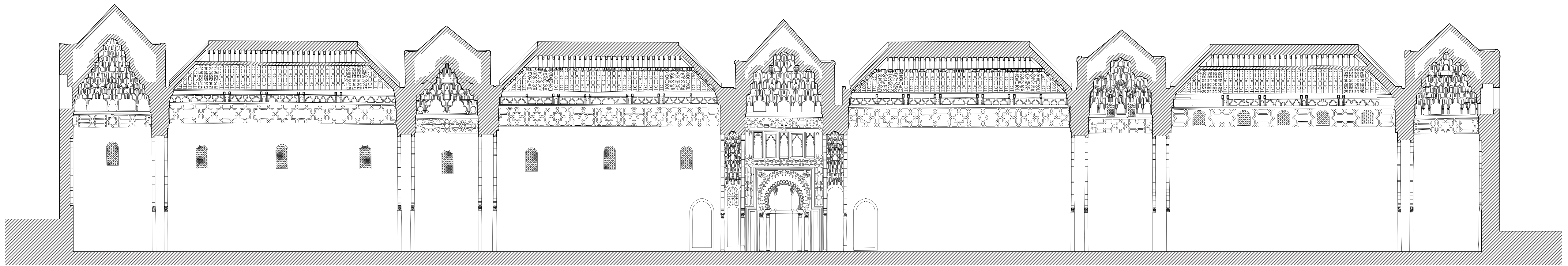
MEZQUITA KUTUBIYYA DE MARRAKECH. SECCIÓN TRANVERSAL POR LA NAVE DE LA QIBLA A. ALMAGRO / ARQ. ESCUELA DE ESTUDIOS ÁRABES, CSIC, GRANADA ENERO 2018
