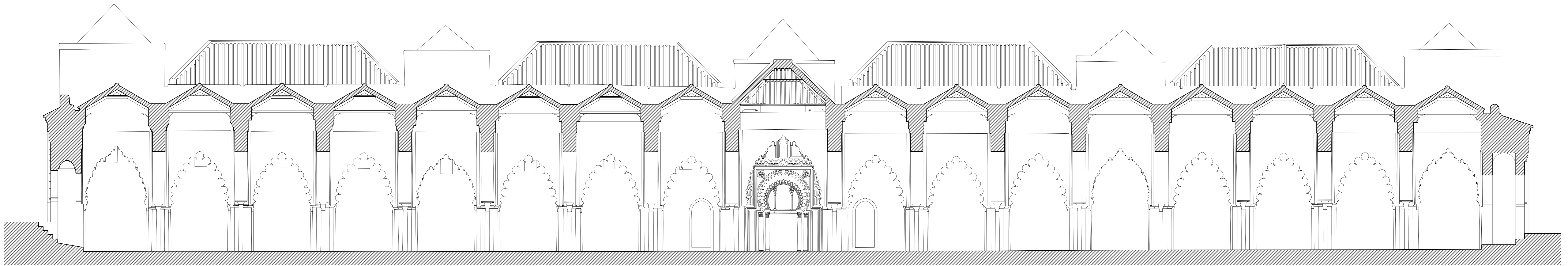
MEZQUITA KUTUBIYYA DE MARRAKECH. SECCIÓN TRANVERSAL POR LA SALA DE ORACION A. ALMAGRO / ARQ. ESCUELA DE ESTUDIOS ÁRABES, CSIC, GRANADA ENERO 2018
