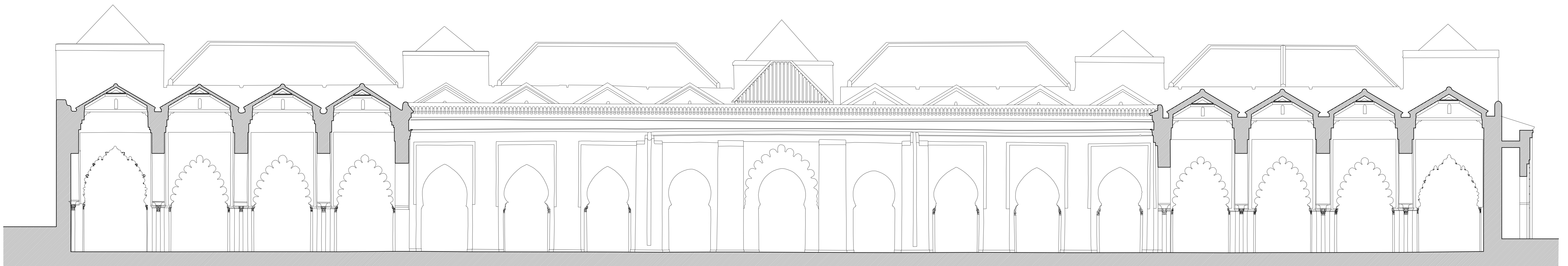
MEZQUITA KUTUBIYYA DE MARRAKECH. SECCIÓN TRANVERSAL POR EL PATIO A. ALMAGRO / ARQ. ESCUELA DE ESTUDIOS ÁRABES, CSIC, GRANADA ENERO 2018
