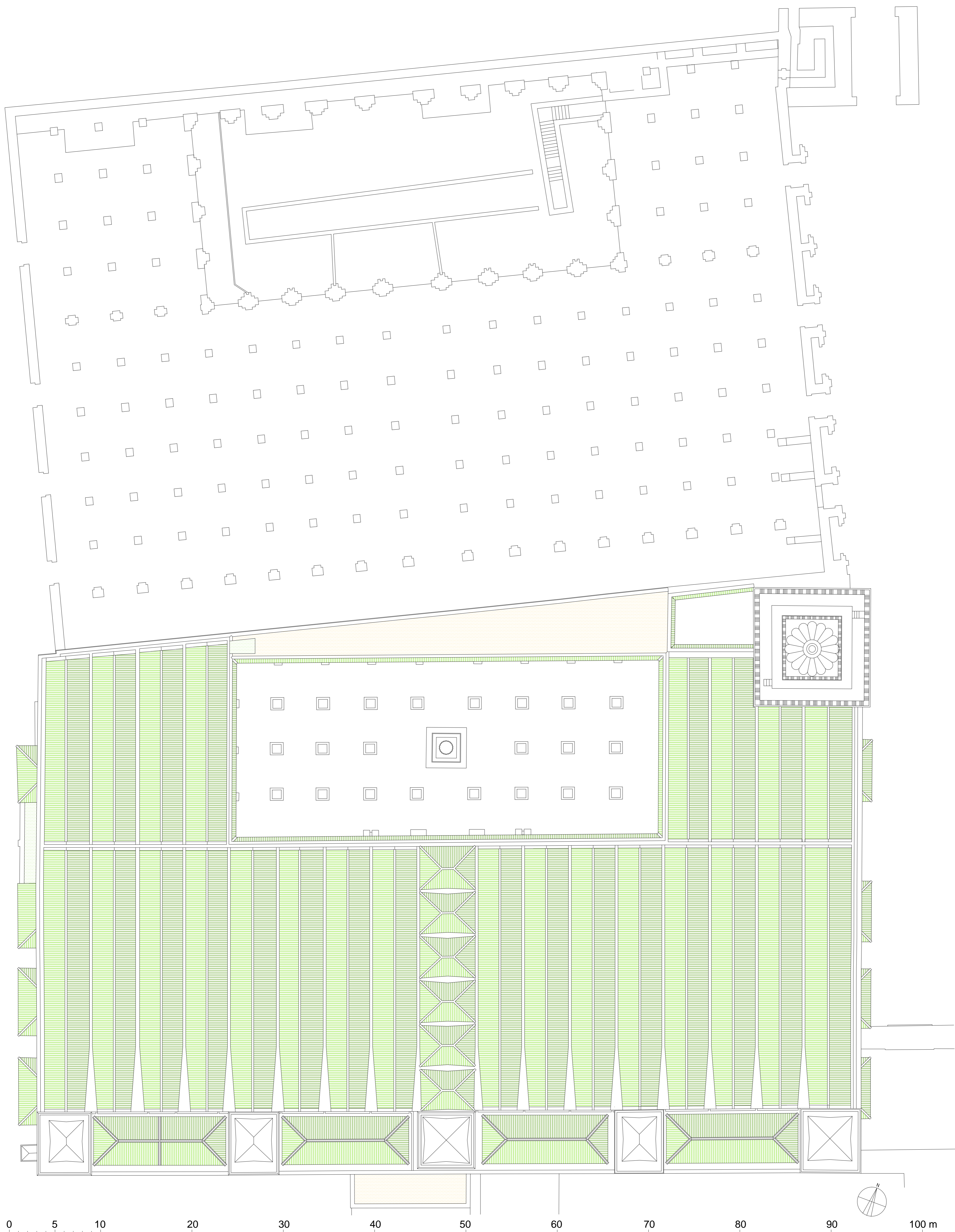
MEZQUITA KUTUBIYYA DE MARRAKECH. PLANTA DE CUBIERTAS.
