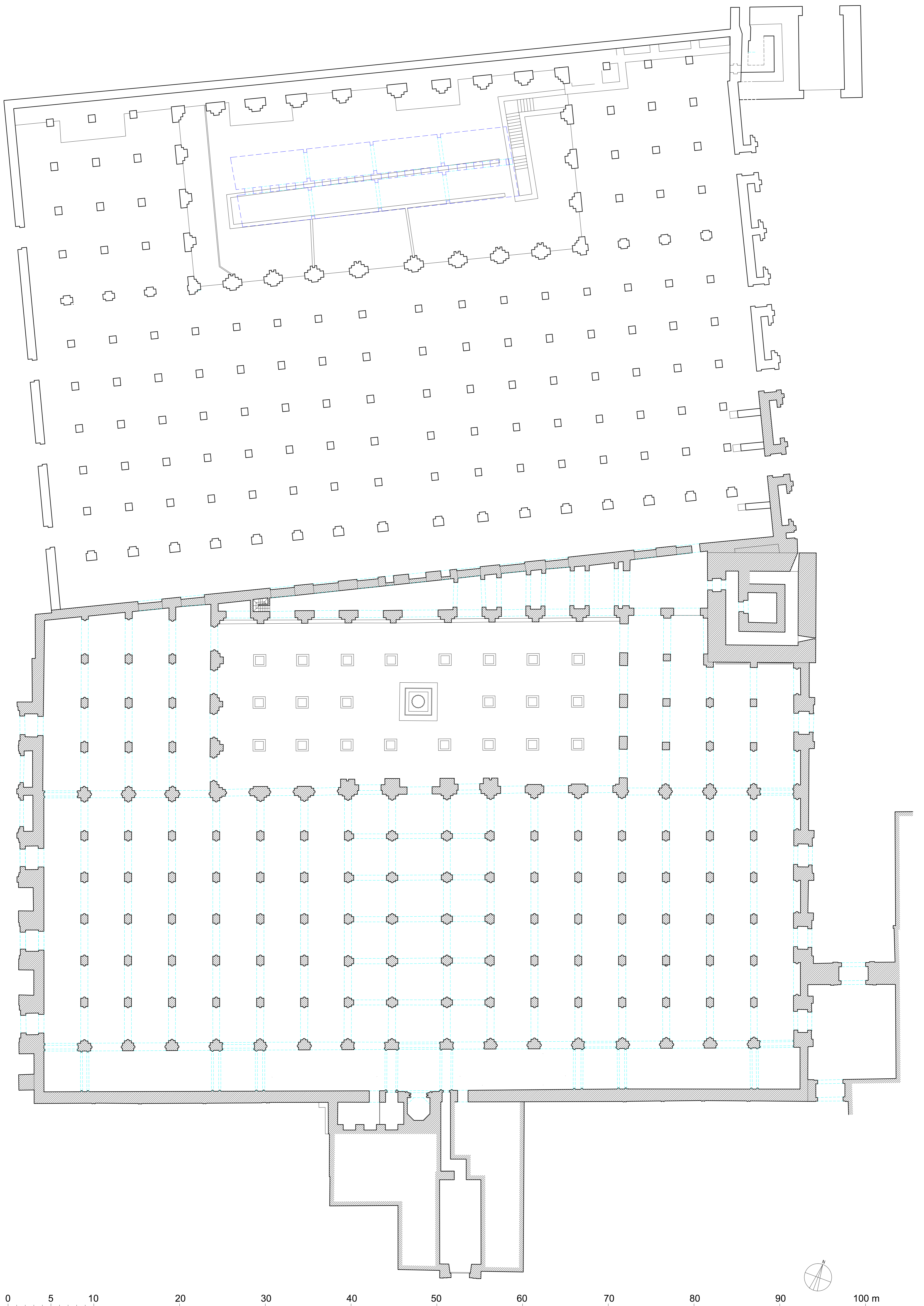
MEZQUITA KUTUBIYYA DE MARRAKECH. PLANTA
