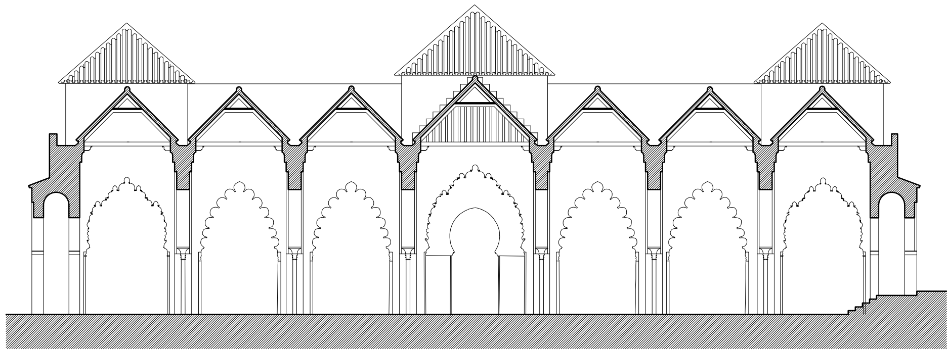
SECCION TRANSVERSAL POR LA SALA DE ORACION
