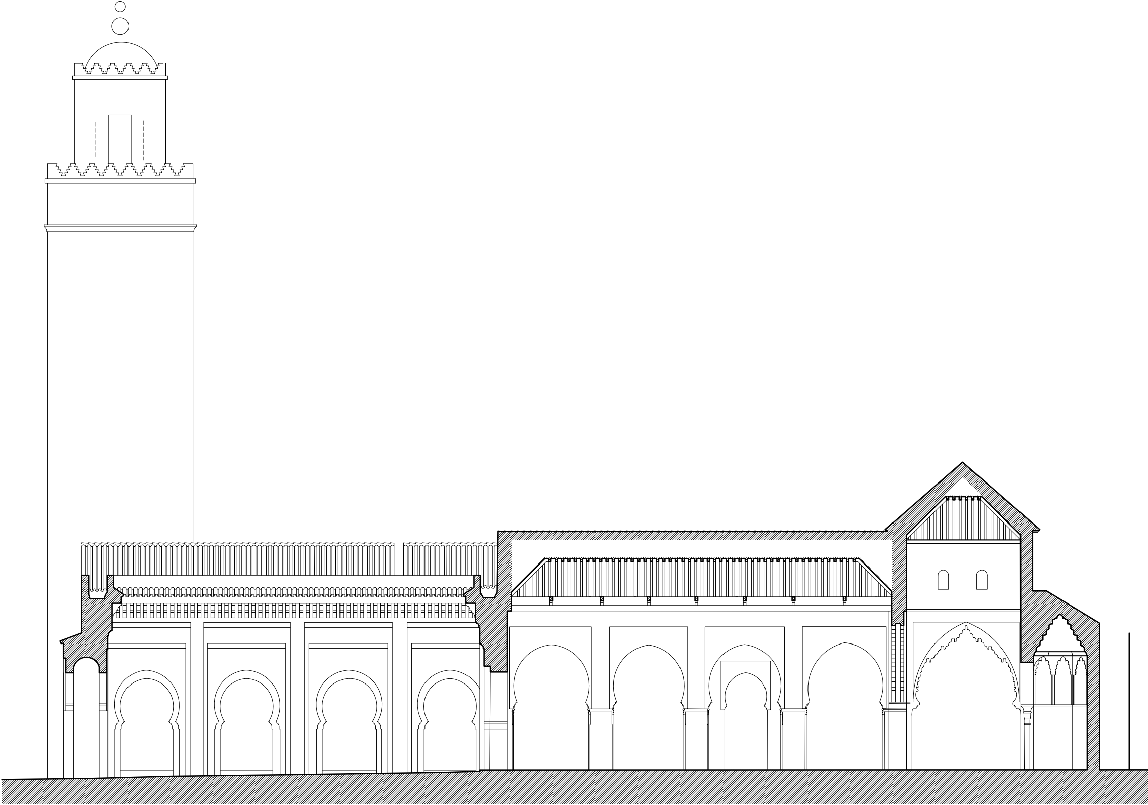
SECCION LONGITUDINAL
