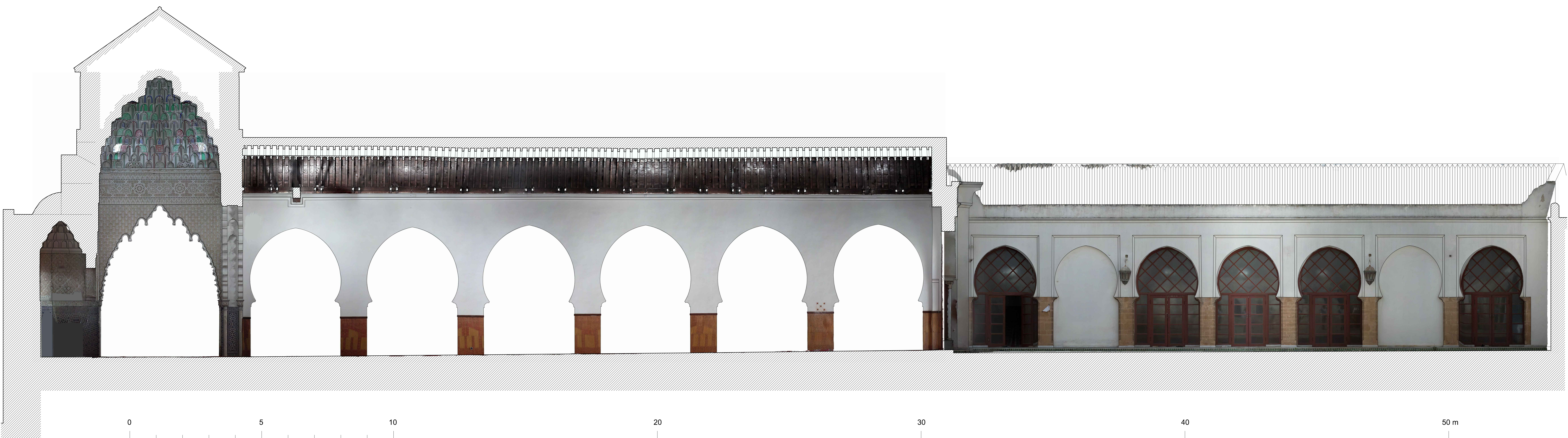
MEZQUITA ALMOHADE DE SALÉ. SECCION LONGITUDINAL POR LA NAVE AXIAL
