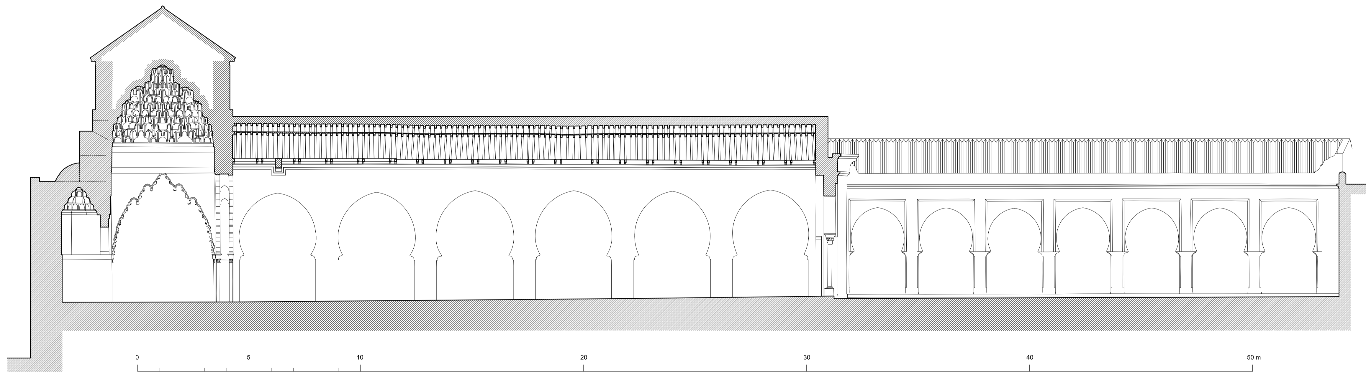
MEZQUITA ALMOHADE DE SALÉ. SECCION LONGITUDINAL POR LA NAVE AXIAL
