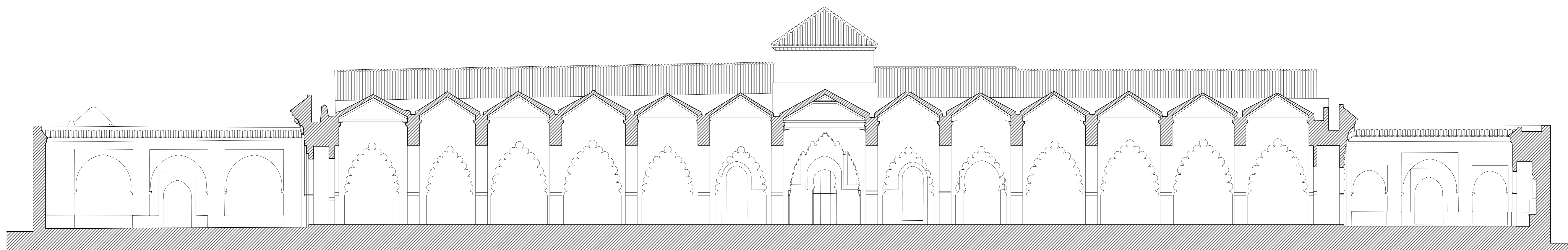
MEZQUITA ALMOHADE DE SALÉ. SECCION POR LA SALA DE ORACION
