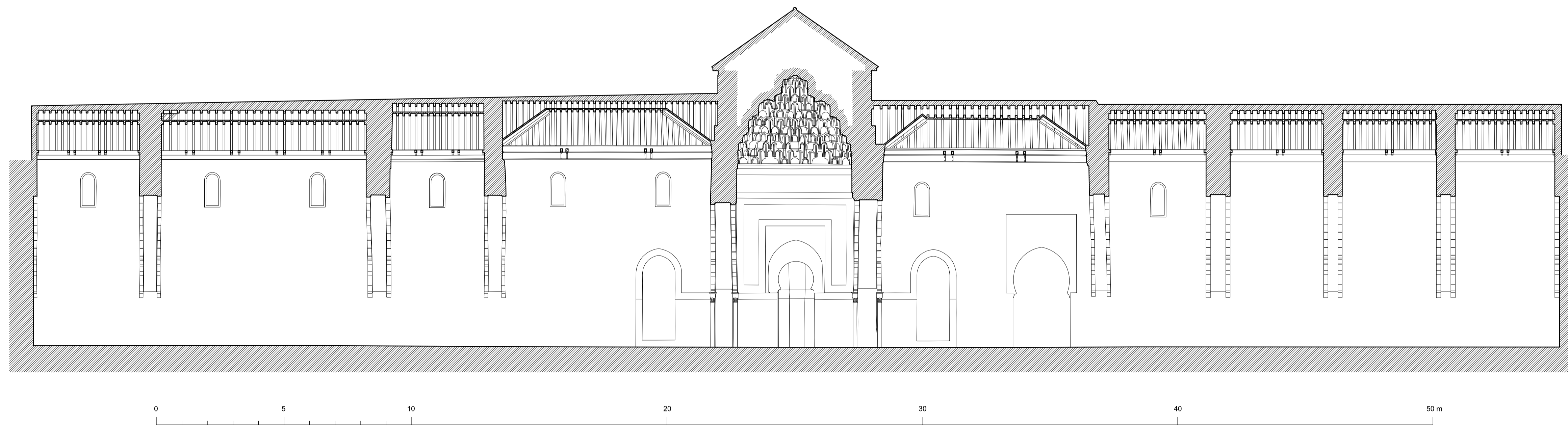
MEZQUITA ALMOHADE DE SALÉ. SECCION POR LA NAVE INMEDIATA AL MURO DE LA QIBLA
