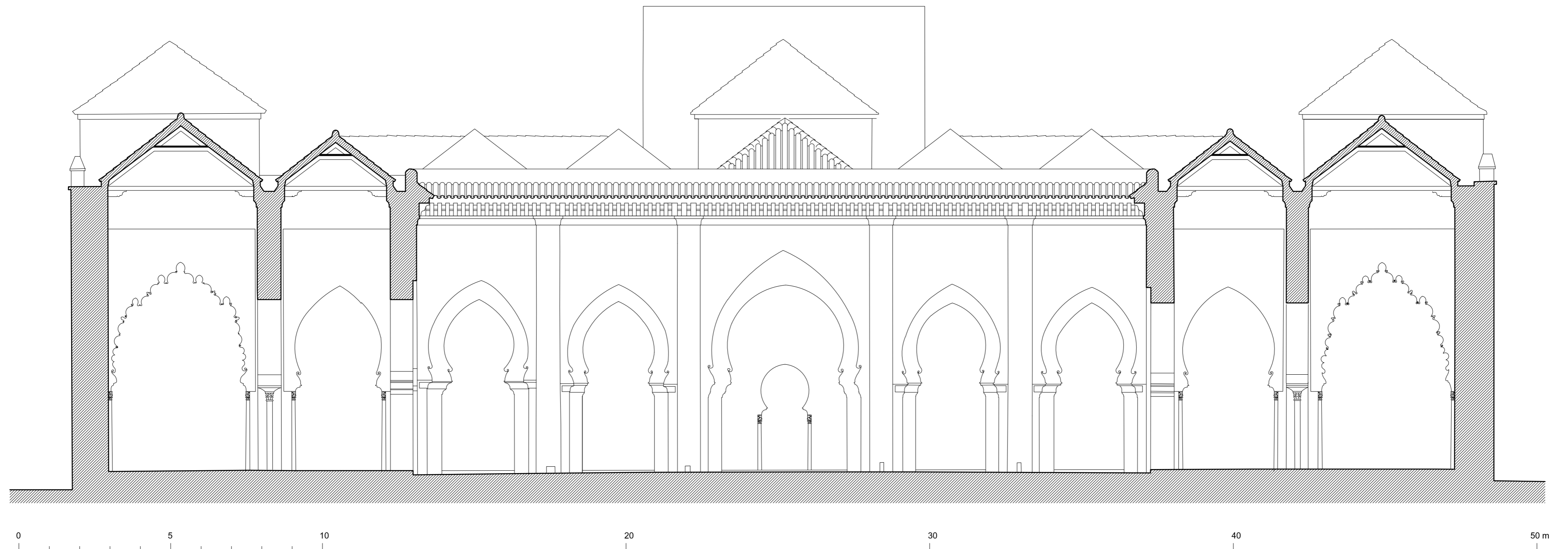
MEZQUITA DE TINMAL. SECCIÓN TRANSVERSAL POR EL PATIO. HIPOTESIS
