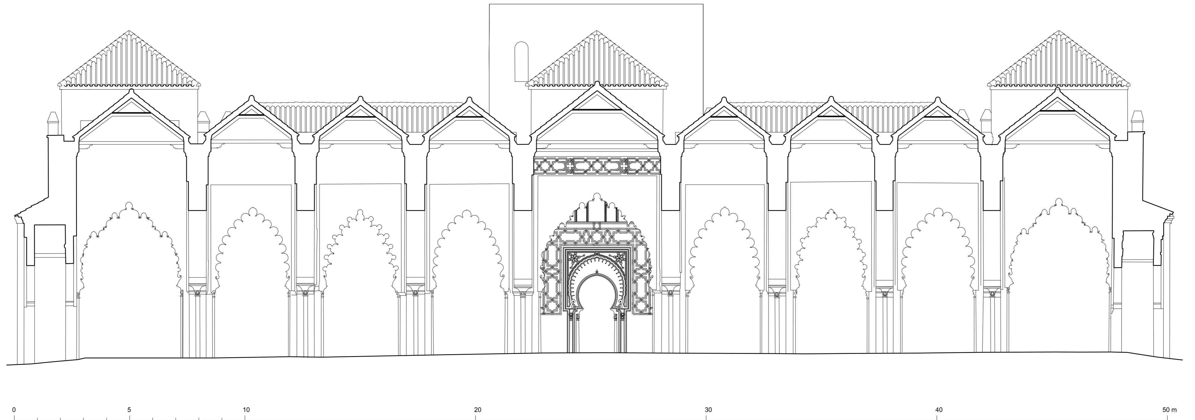
MEZQUITA DE TINMAL. SECCIÓN TRANSVERSAL POR LA SALA DE ORACIÓN. HIPÓTESIS
