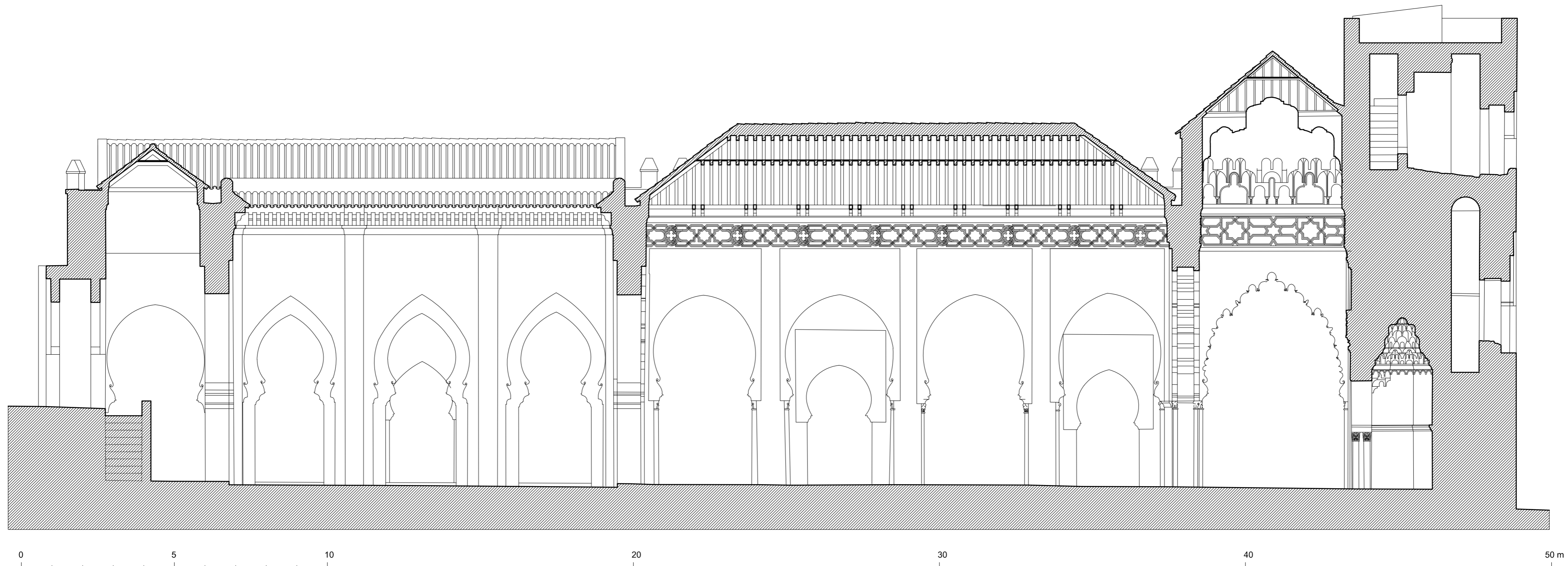
MEZQUITA DE TINMAL. SECCIÓN LONGITUDINAL POR LA NAVE CENTRAL. HIPÓTESIS
