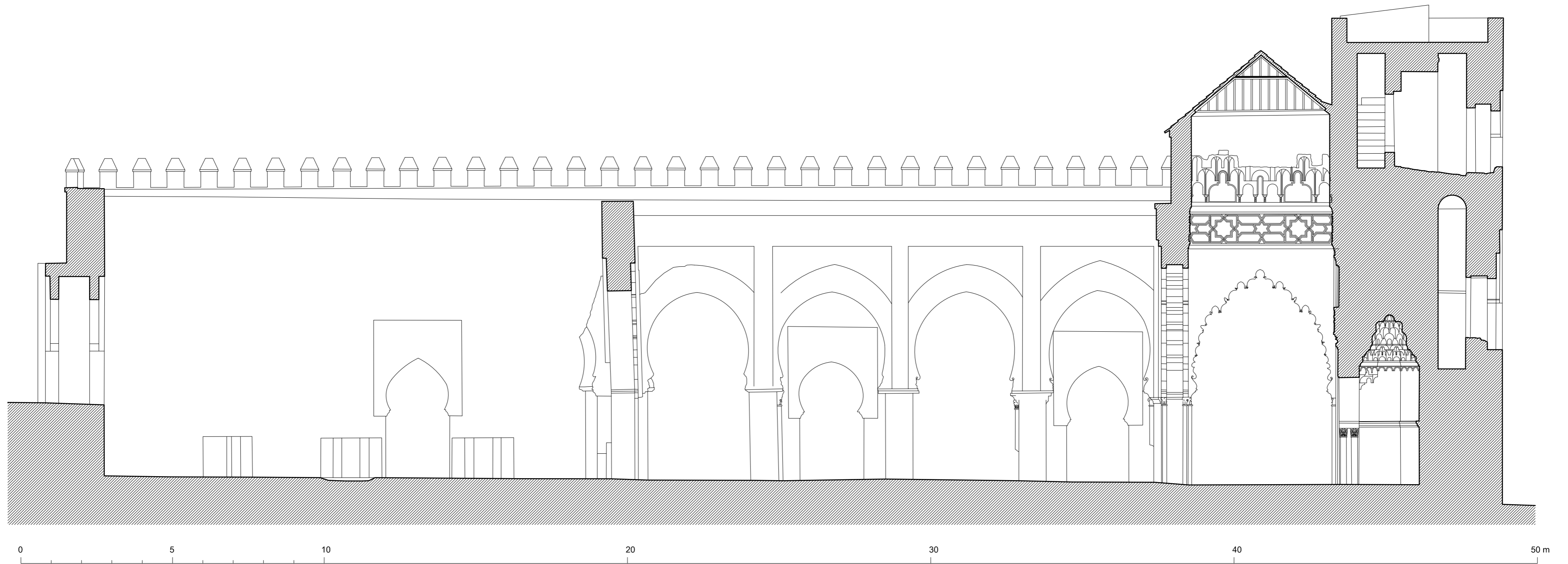
MEZQUITA DE TINMAL. SECCIÓN LONGITUDINAL POR LA NAVE CENTRAL
