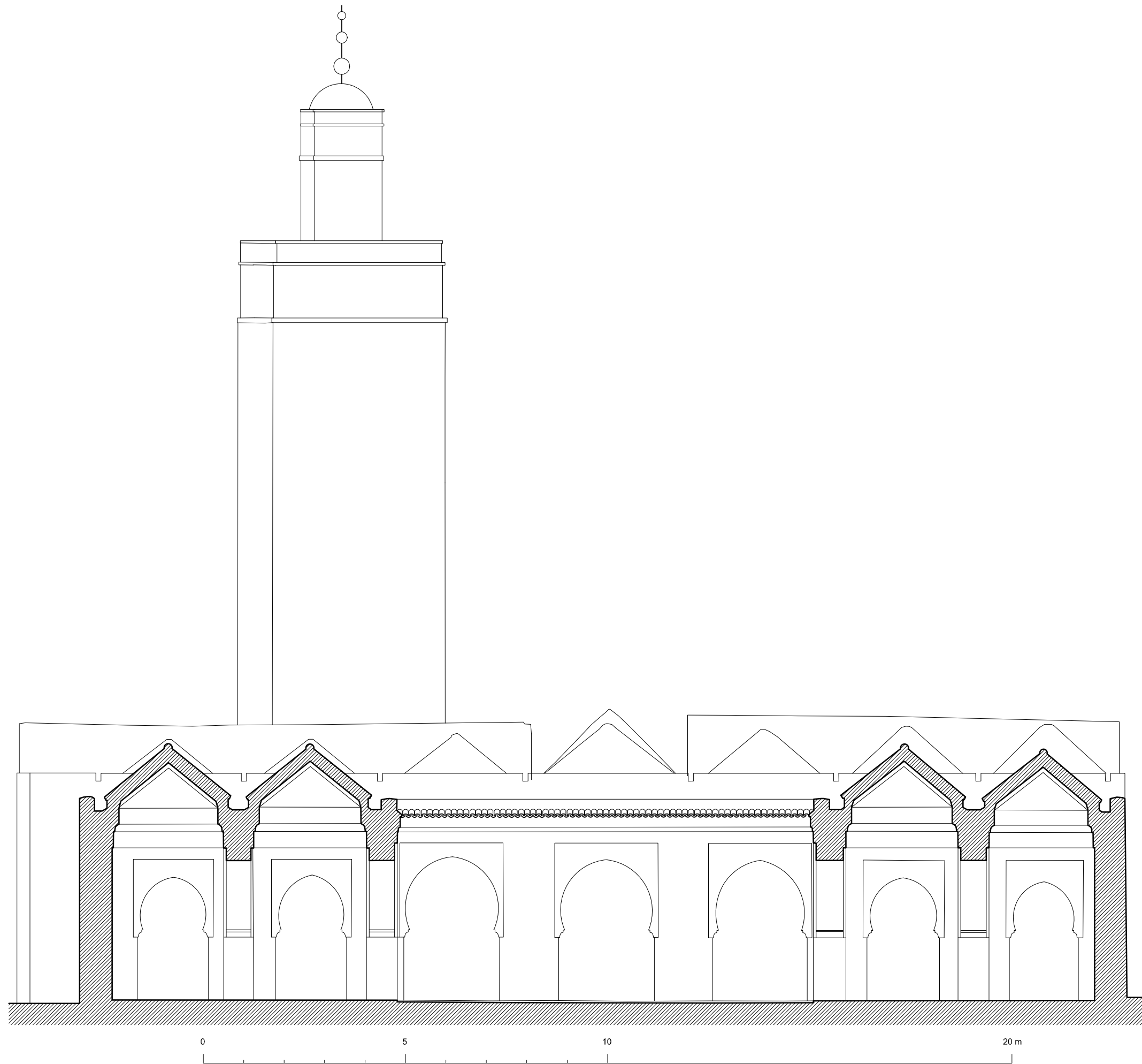
MEZQUITA AL-ATIQU EN LA QASBA DE RABAT. SECCION TRANSVERSAL POR EL PATIO. HIPOTESIS
