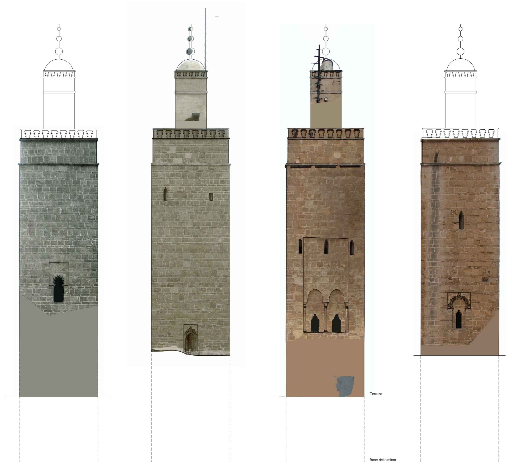
ALZADO NOROESTE
