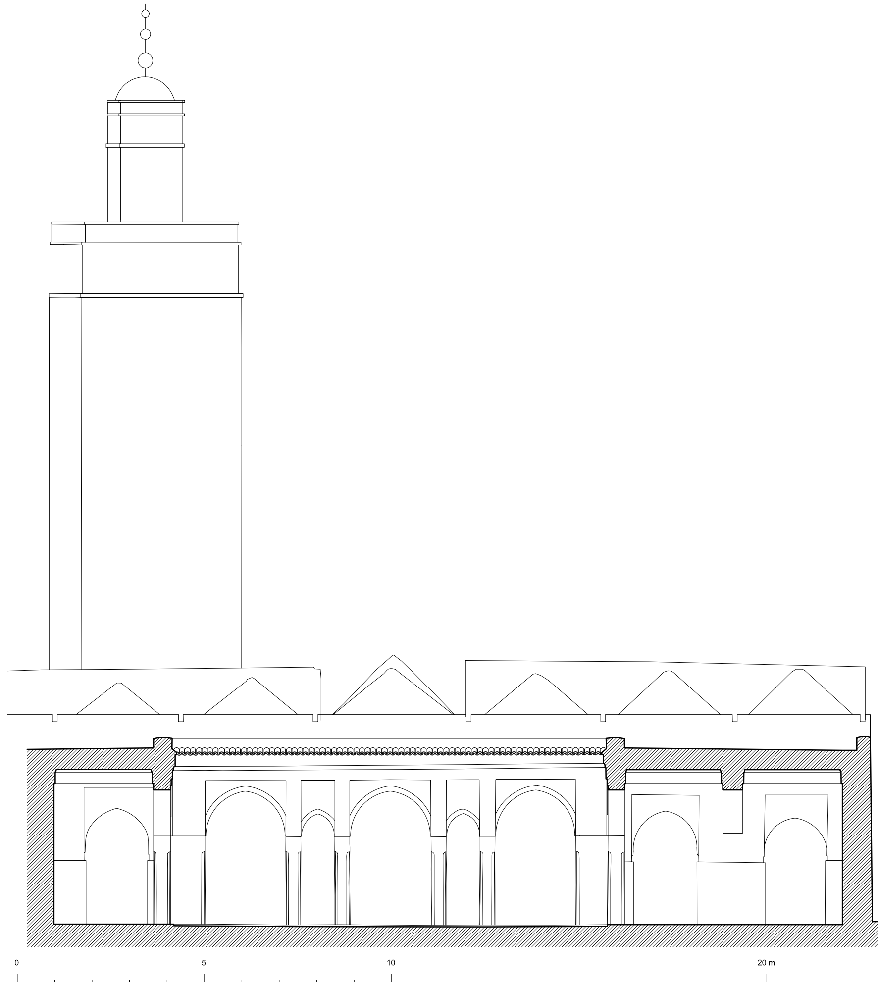
MEZQUITA AL-ATIQU EN LA QASBA DE RABAT. SECCION TRANSVERSAL POR EL PATIO
