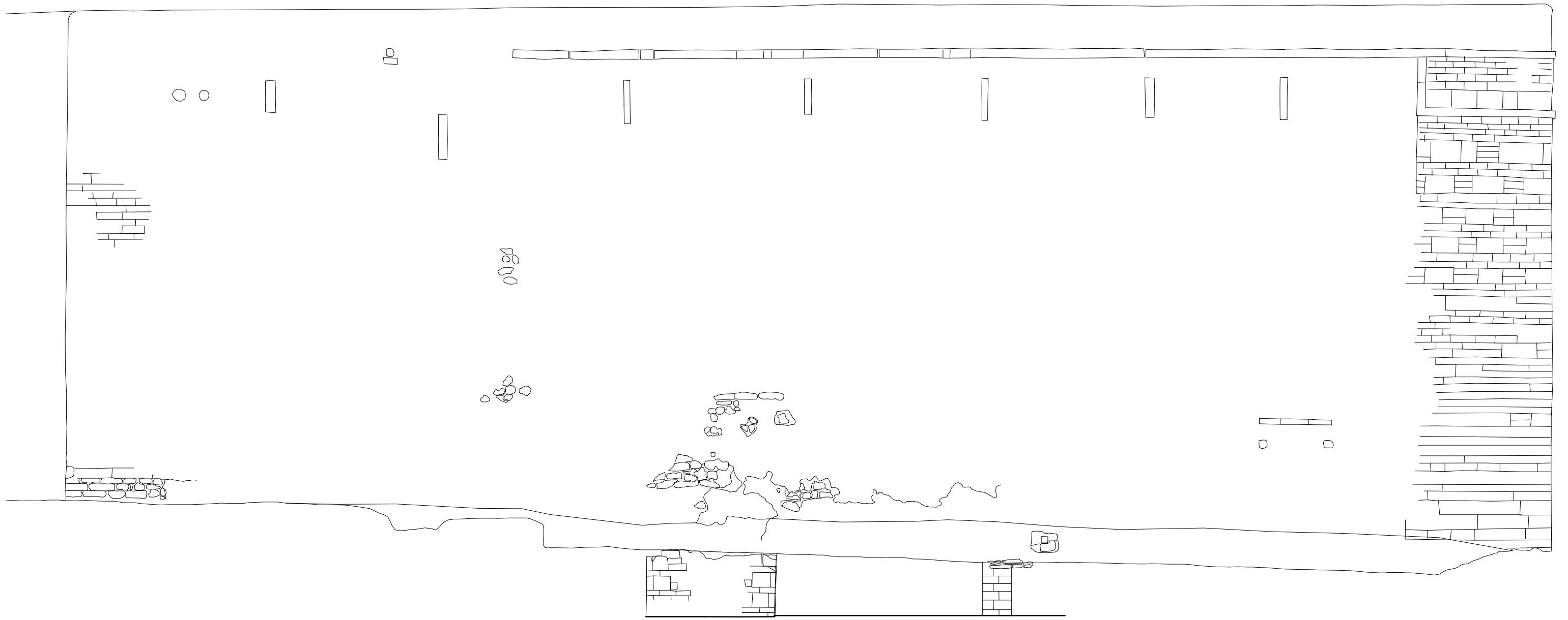
QASBA DE RABAT. BAB AL-KEBIR. ALZADO EXTERIOR. ANTONIO ALMAGRO. ESCUELA DE STUDIOS ARABES, CSIC. GRANADA.
