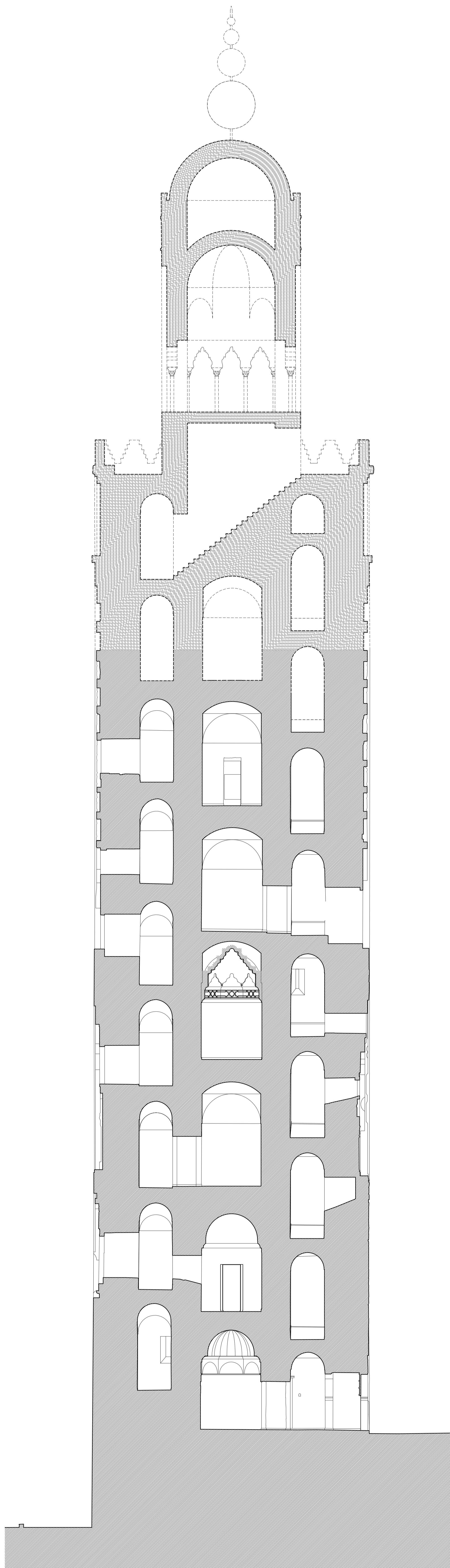
ALMINAR DE LA MEZQUITA ALMOHADE DE RABAT. SECCION N-S
