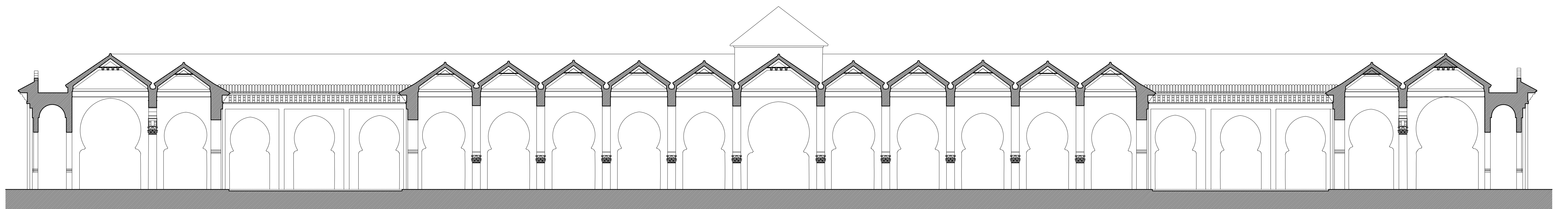
0 5 10 20 30 40 50 m MEZQUITA ALMOADE DE RABAT. SECCION TRANSVERSAL POR LOS PATOS MENORES A. ALMORREI ARZ. RABAT FEBRERO 2021
