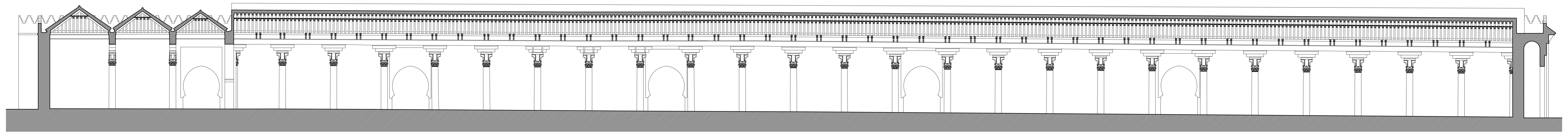
MEZQUITA ALMORÁVIDE DE RABAT. SECCIÓN LONGITUDINAL JUNTO AL MURO OESTE A. ALVARADO - IREB - FEBRERO 2011
