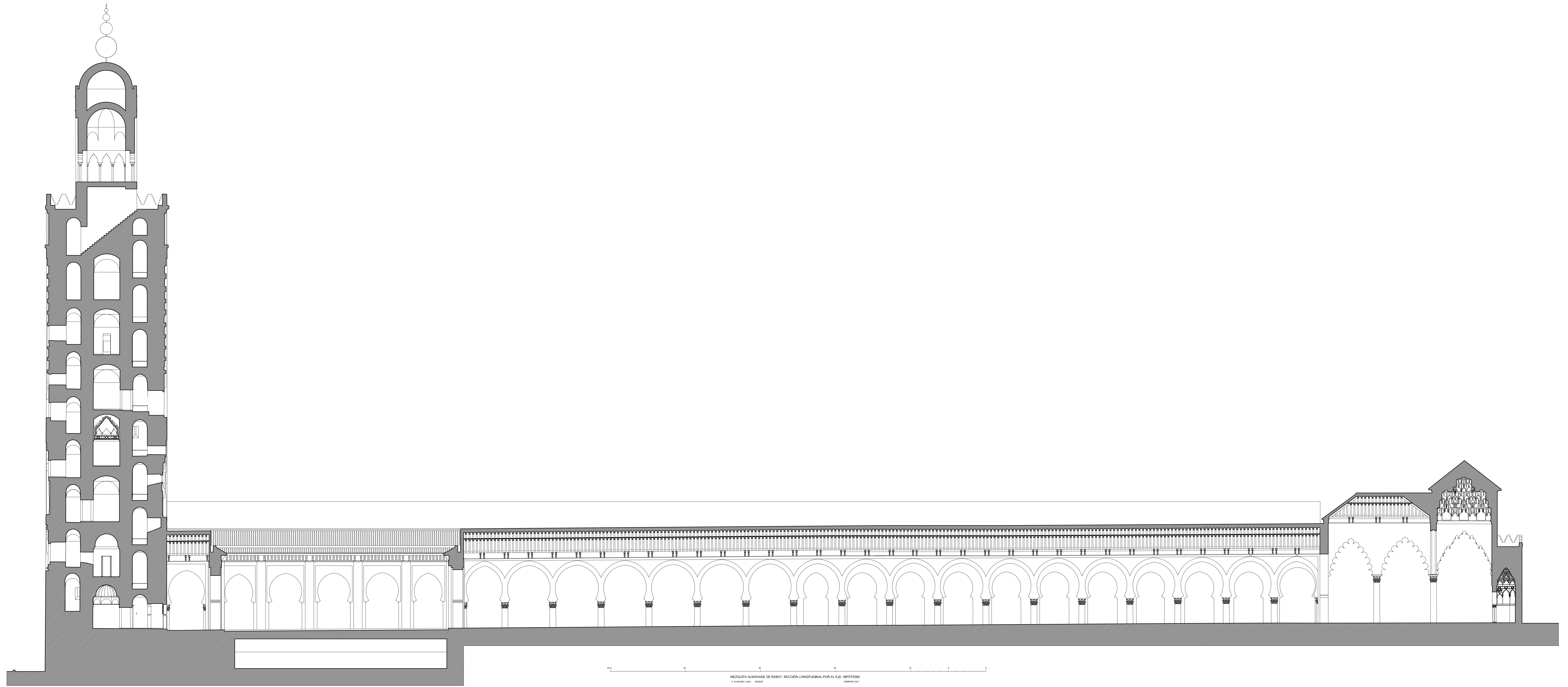
MEZQUITA AL-MOHAR DE MARAT. SECCION LONGITUDINAL POR EL E.E. HIPOTESIS
