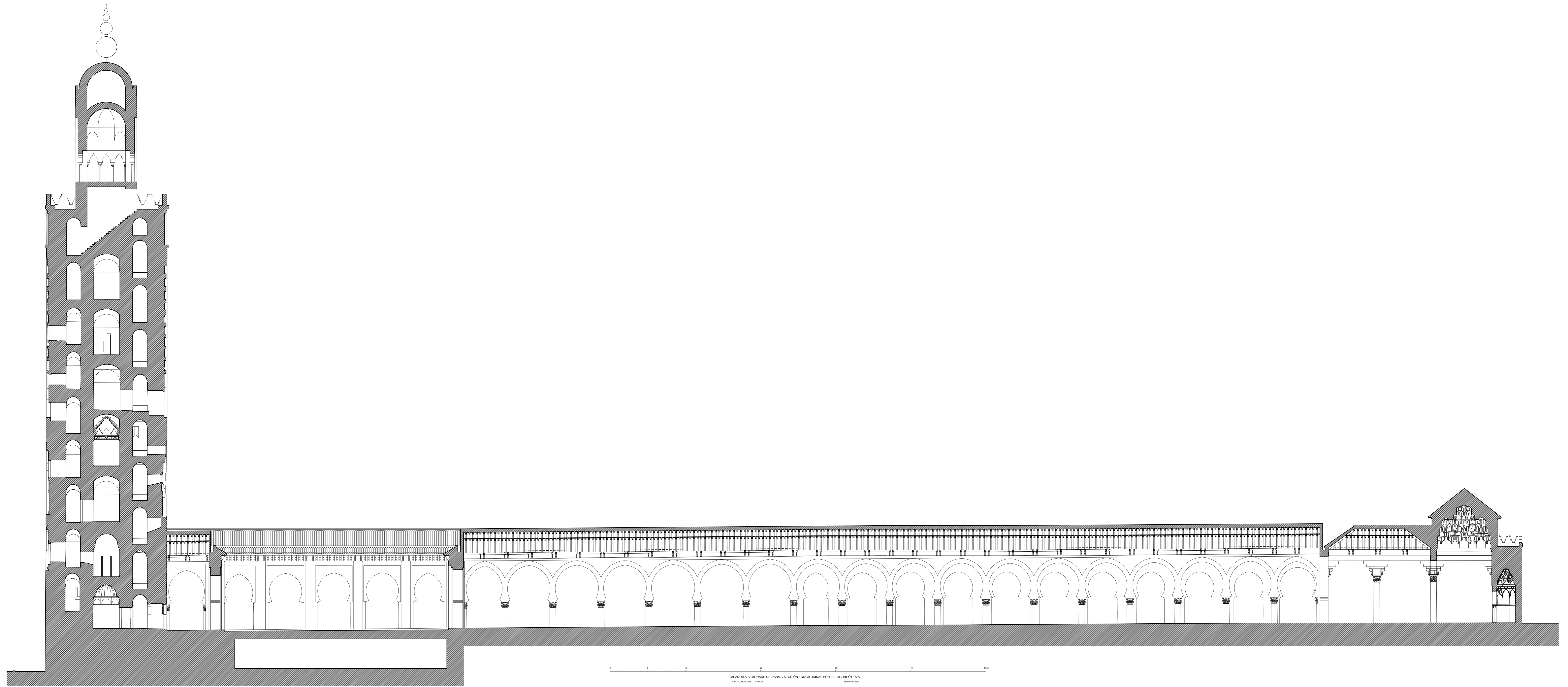
MEZQUITA ALMORHADE DE MARRAKECH. SECCION LONGITUDINAL POR EL E.E. HIPOTESIS
