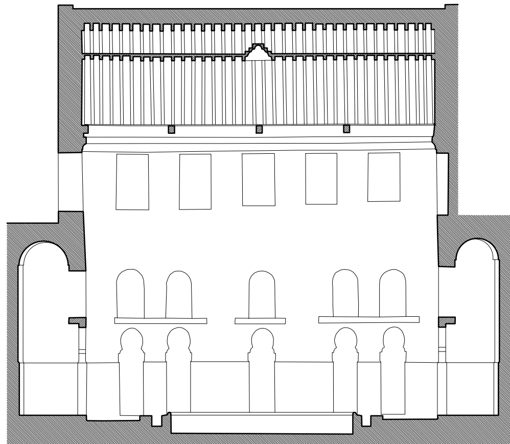
SECCIÓN LONGITUDINAL
