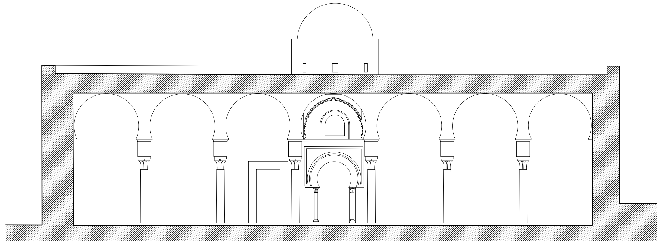
SECCION TRANSVERSAL
