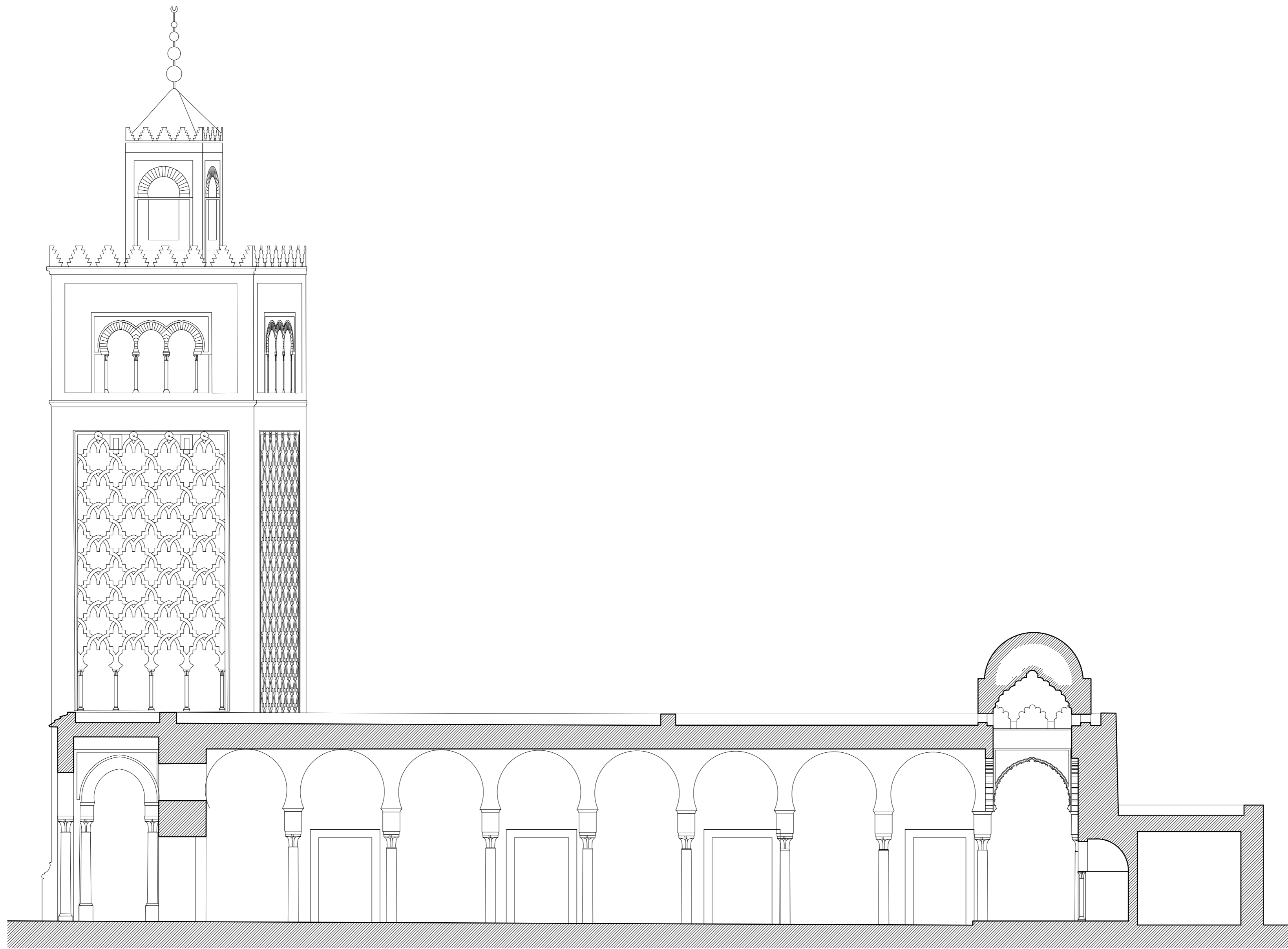
SECCION LONGITUDINAL
