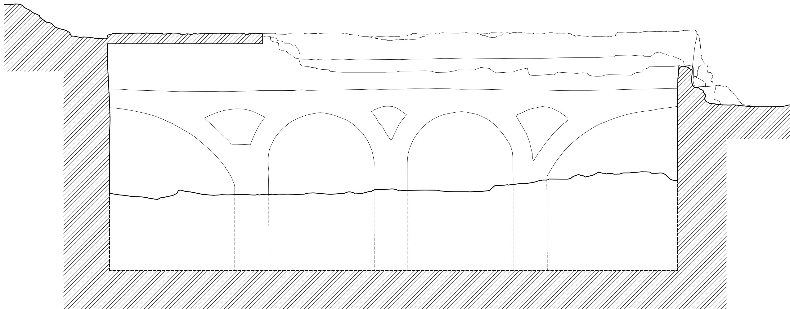
SECCION LONGITUDINAL
