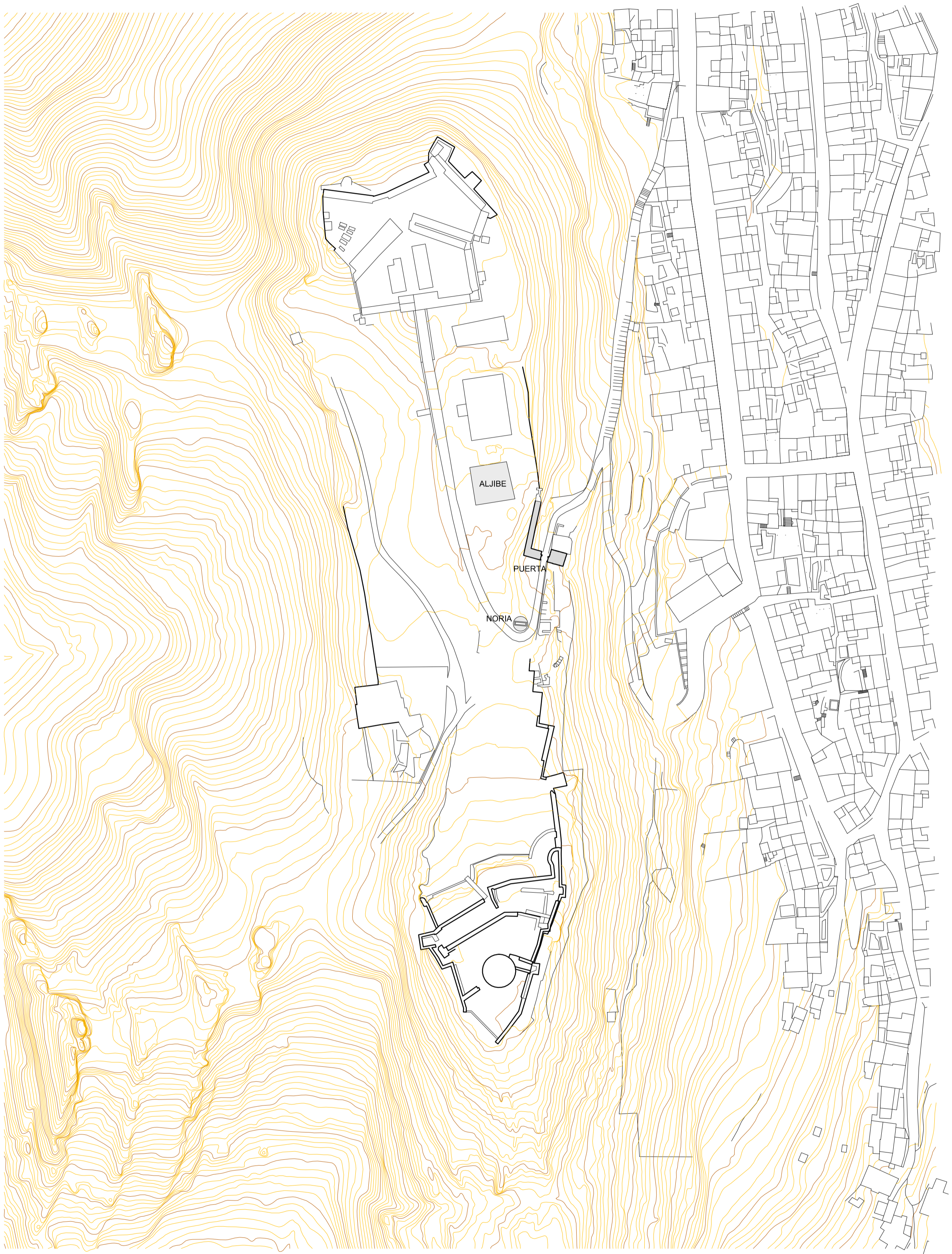
CASTILLO DE JIMENA DE LA FRONTERA (CADIZ). PLANTA GENERAL A. ALMAGRO / arq. RABASF JULIO 2023
