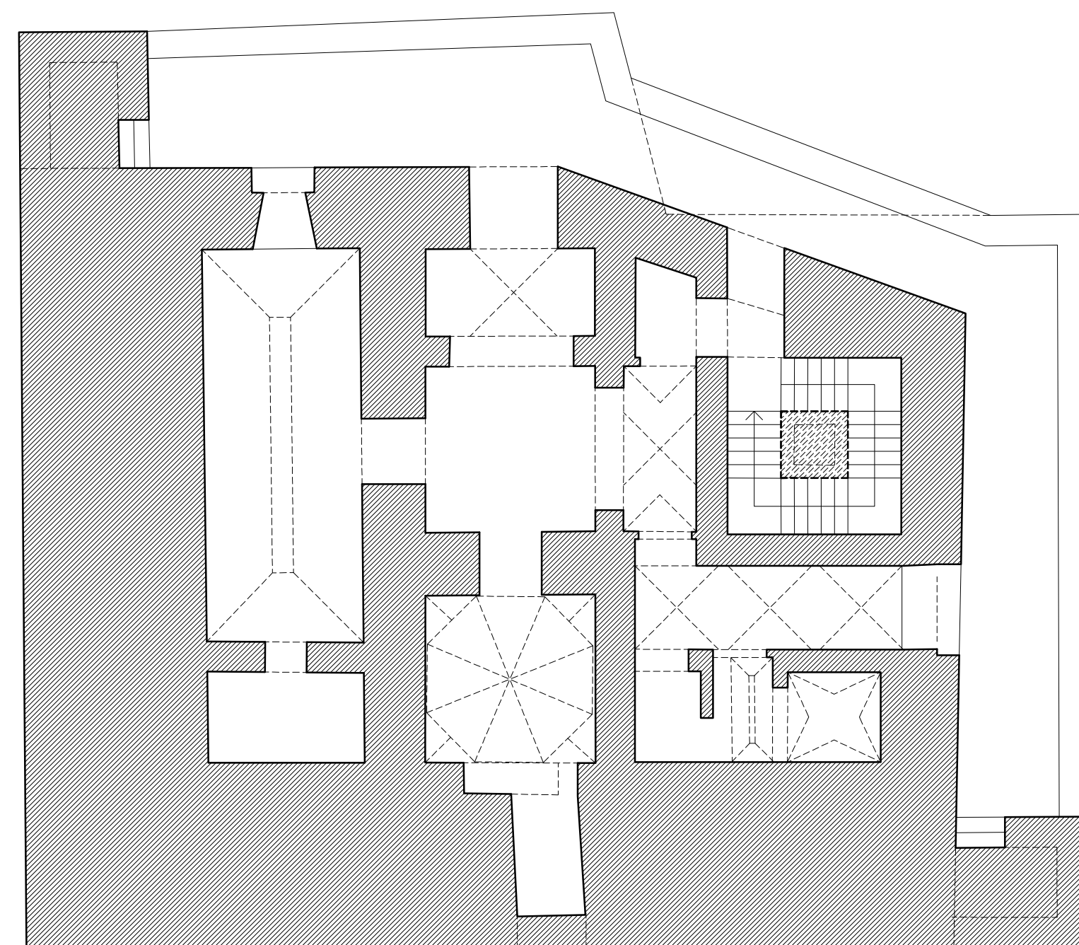
PLANTA NIVEL DE VIVIENDA
