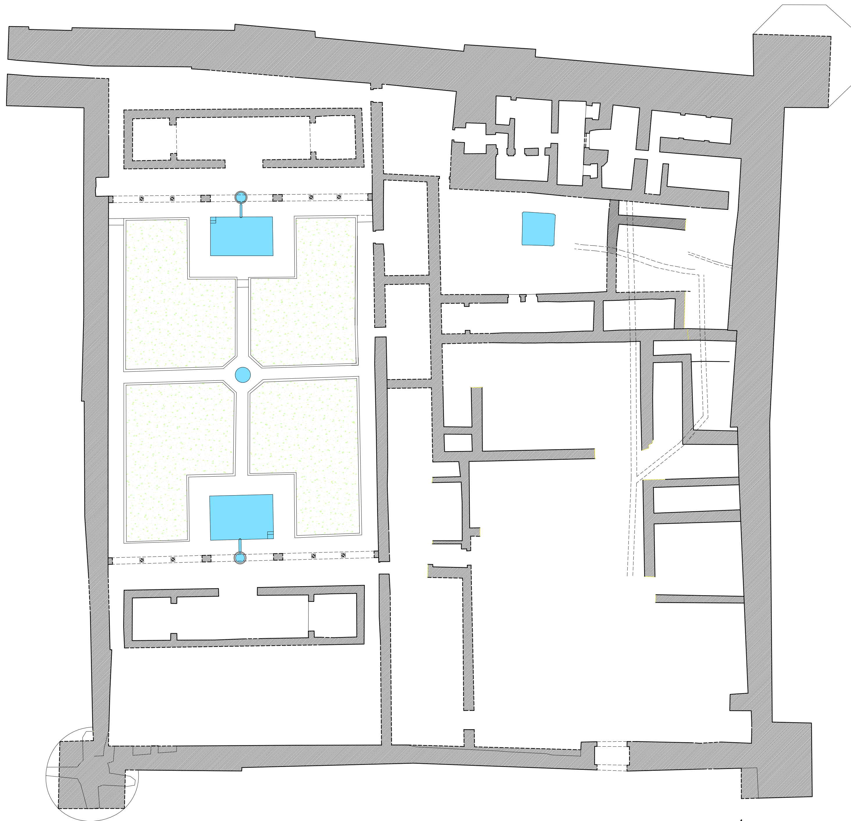
ALCAZAR DE CORDOBA. PALACIO ALMOHADE. Planta hipótesis
