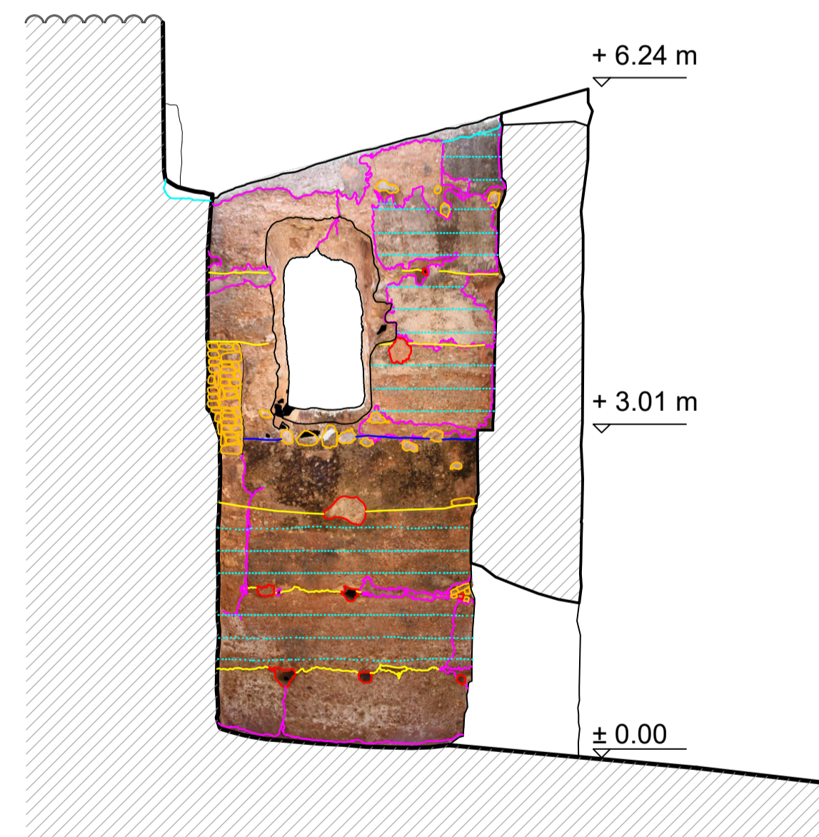
CARA INTERIOR OESTE (2-2')
