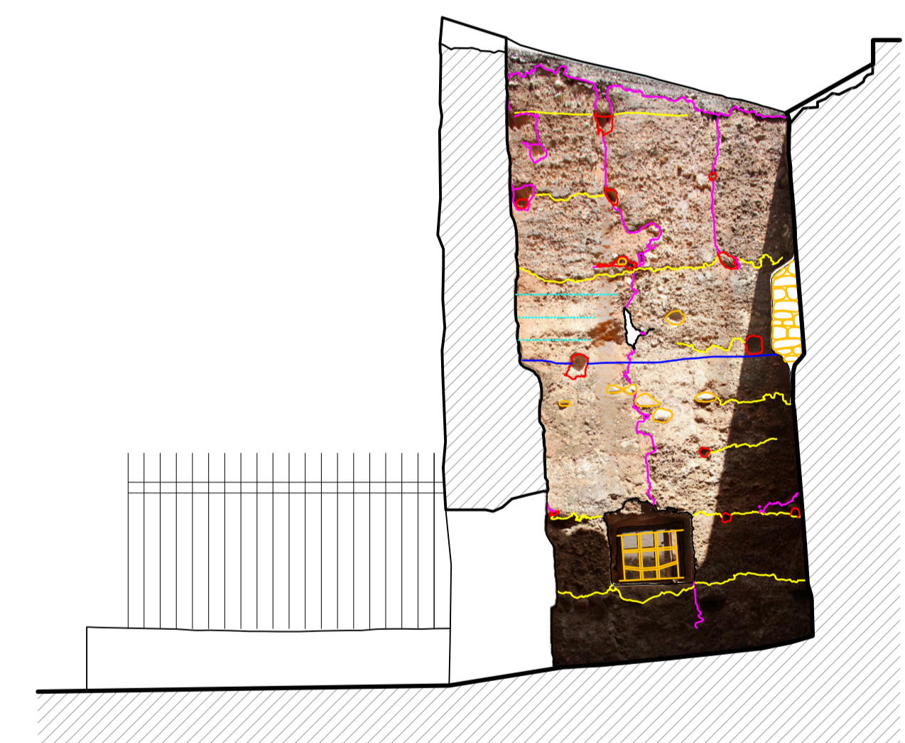
CARA INTERIOR ESTE (4-4')
