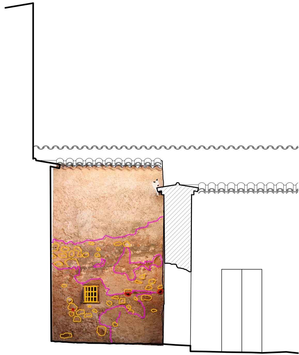
CARA SUR (A-A)
