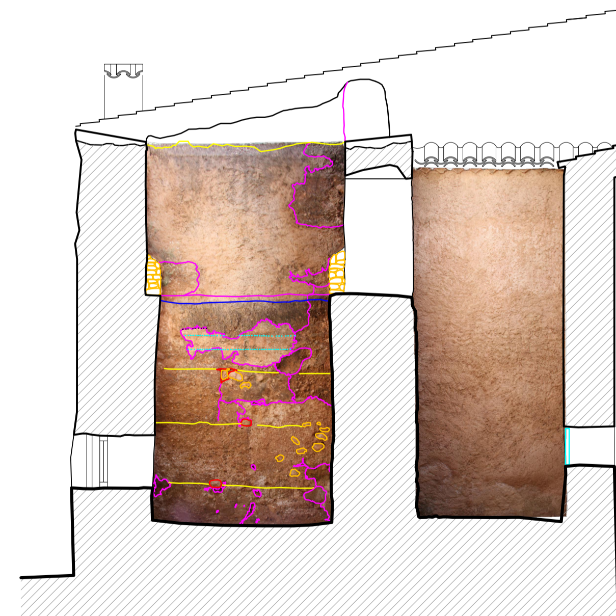
CARA INTERIOR SUR (3-3')
