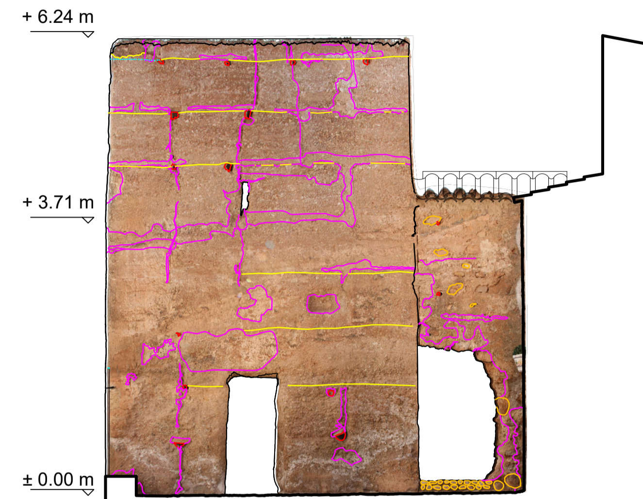
CARA NORTE (C-C')
