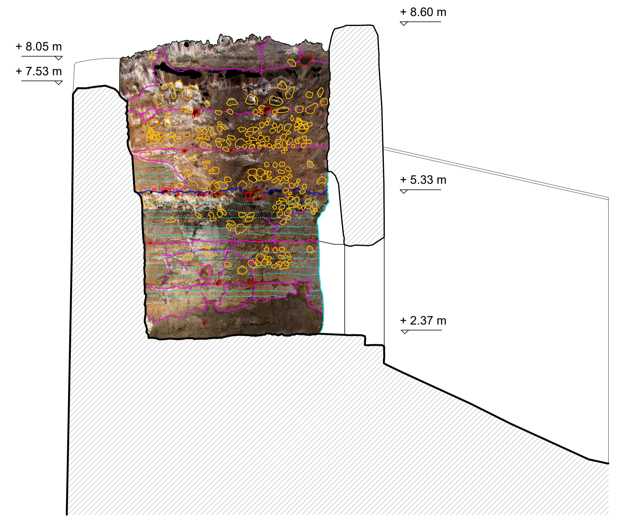
ALZADO INTERIOR NORTE (2-2')
