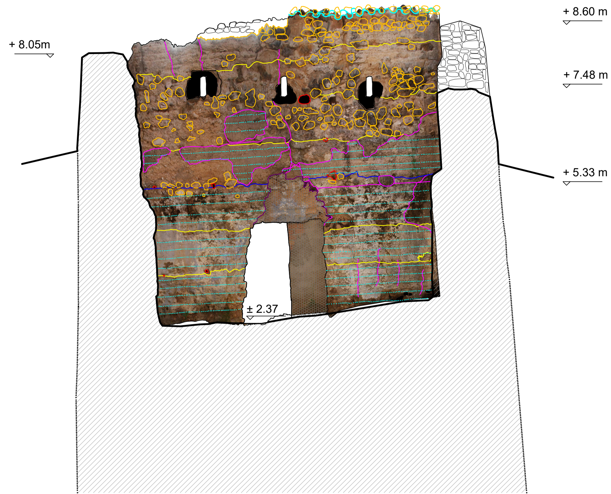
ALZADO INTERIOR ESTE (1-1')
