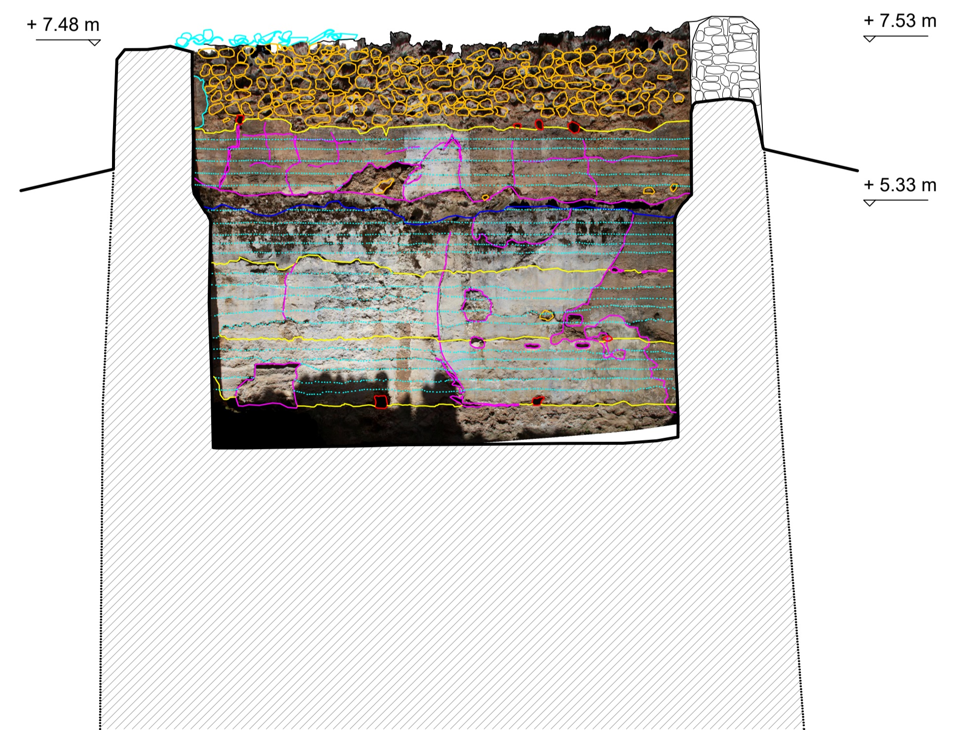
ALZADO INTERIOR OESTE (4-4')
