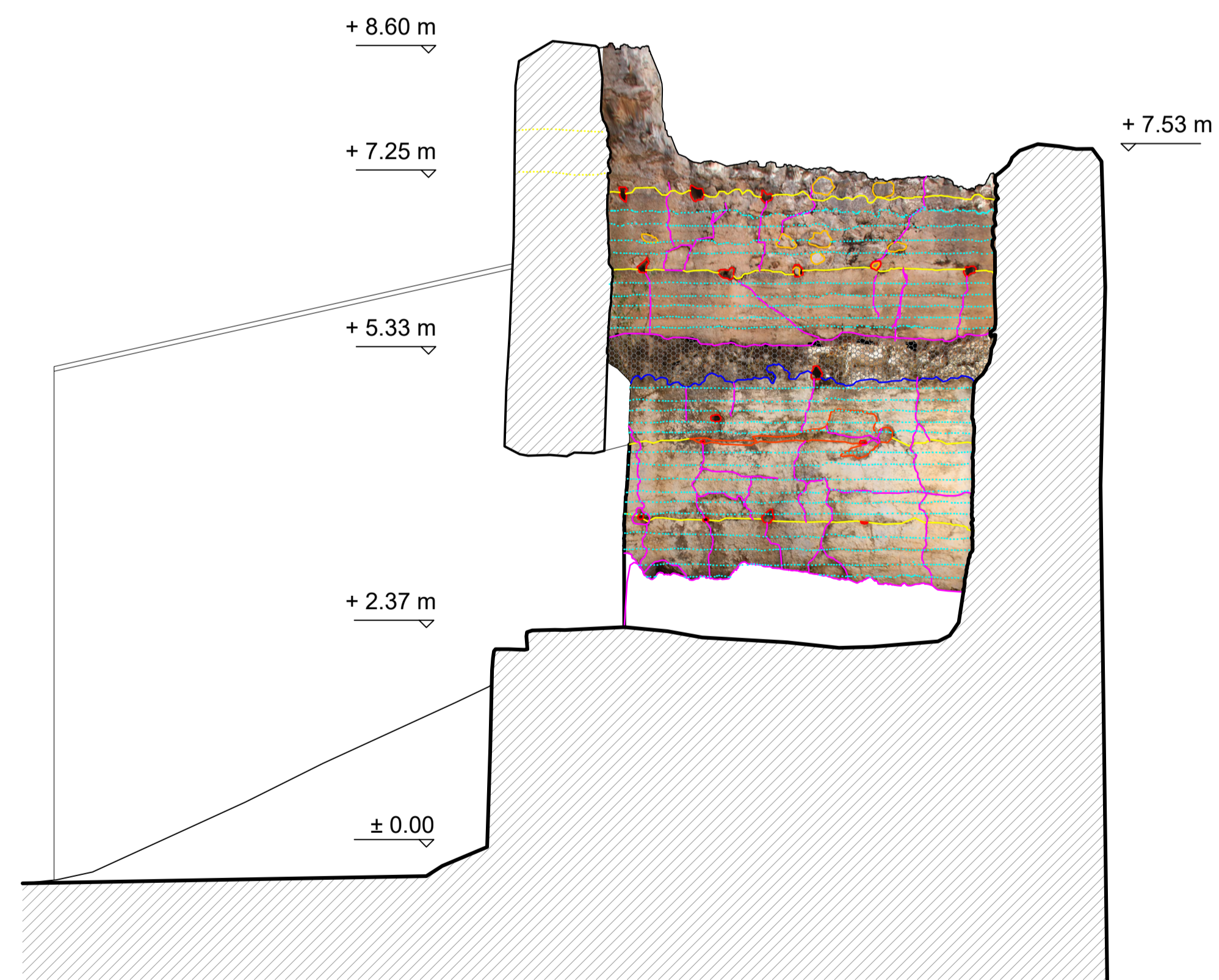
ALZADO INTERIOR SUR (3-3')
