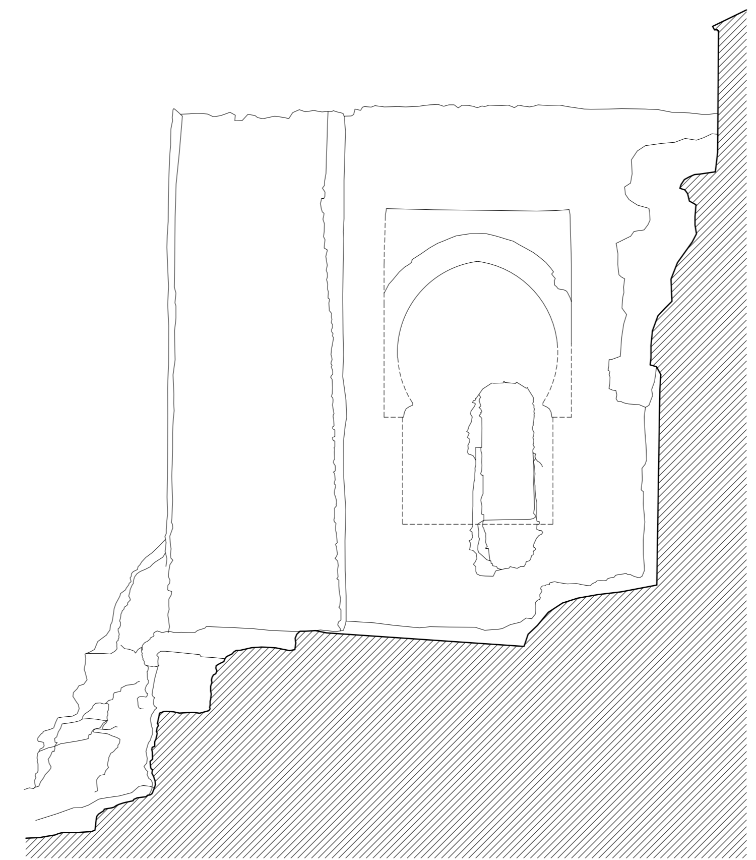
ALZADO SUROCCIDENTE
